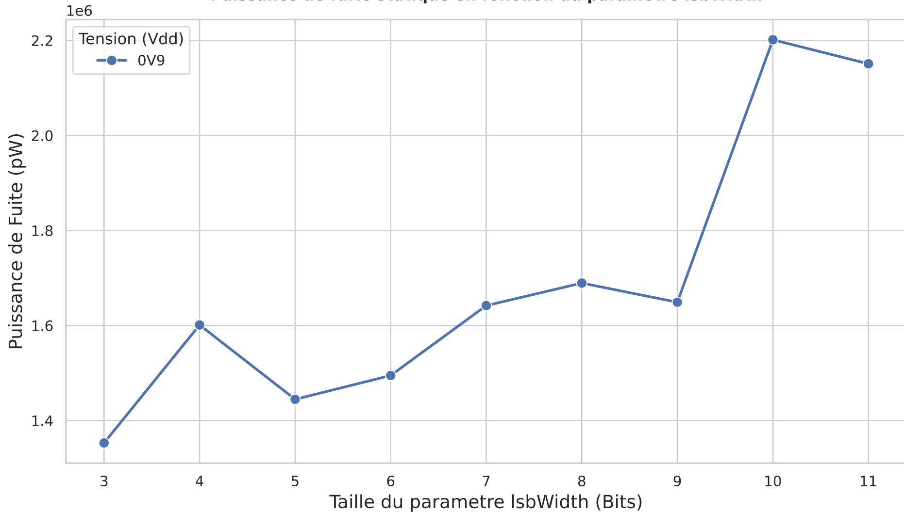
Puissance de fuite statique en fonction du parametre lsbWidth
