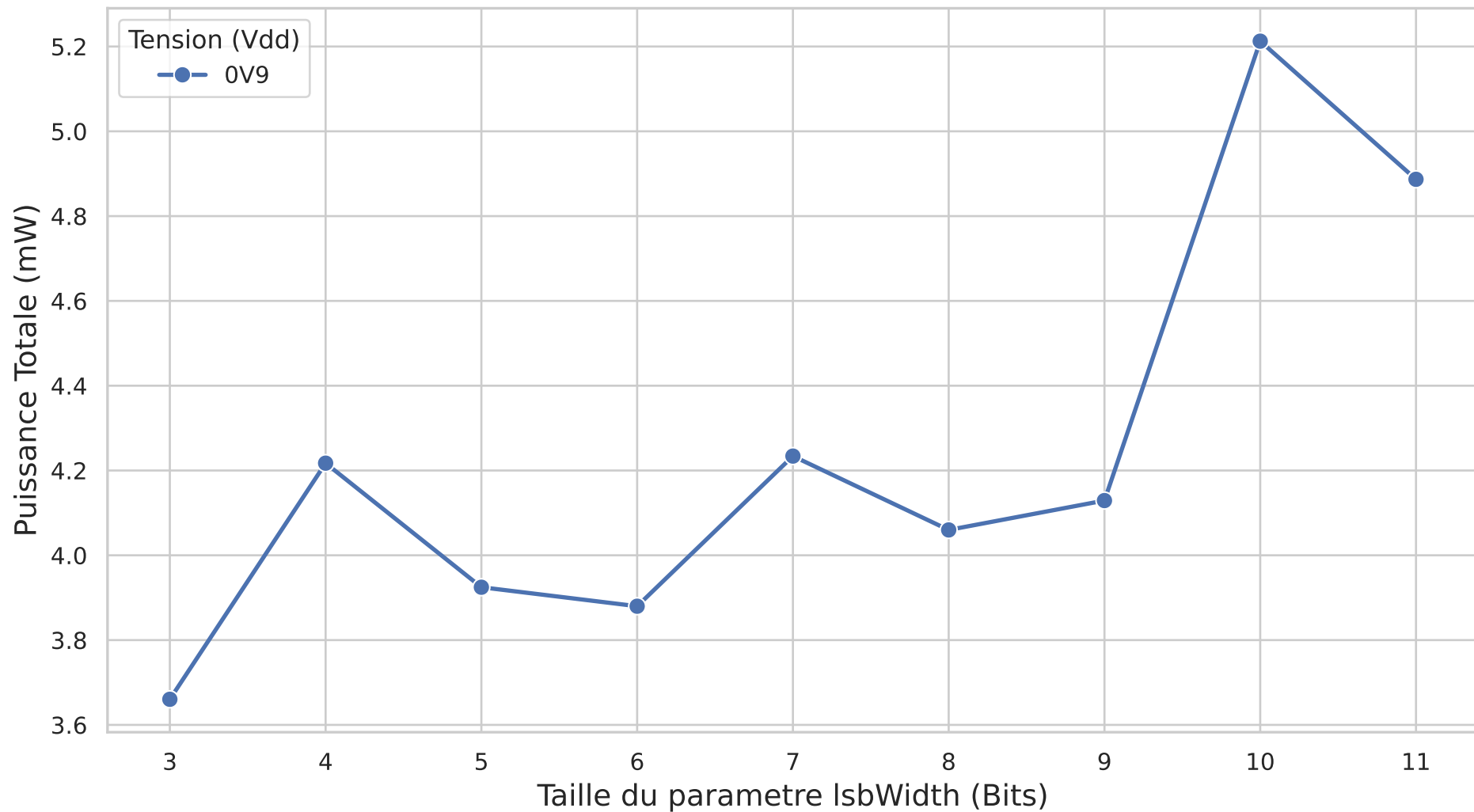
Consommation energetique totale en fonction du parametre lsbWidth
