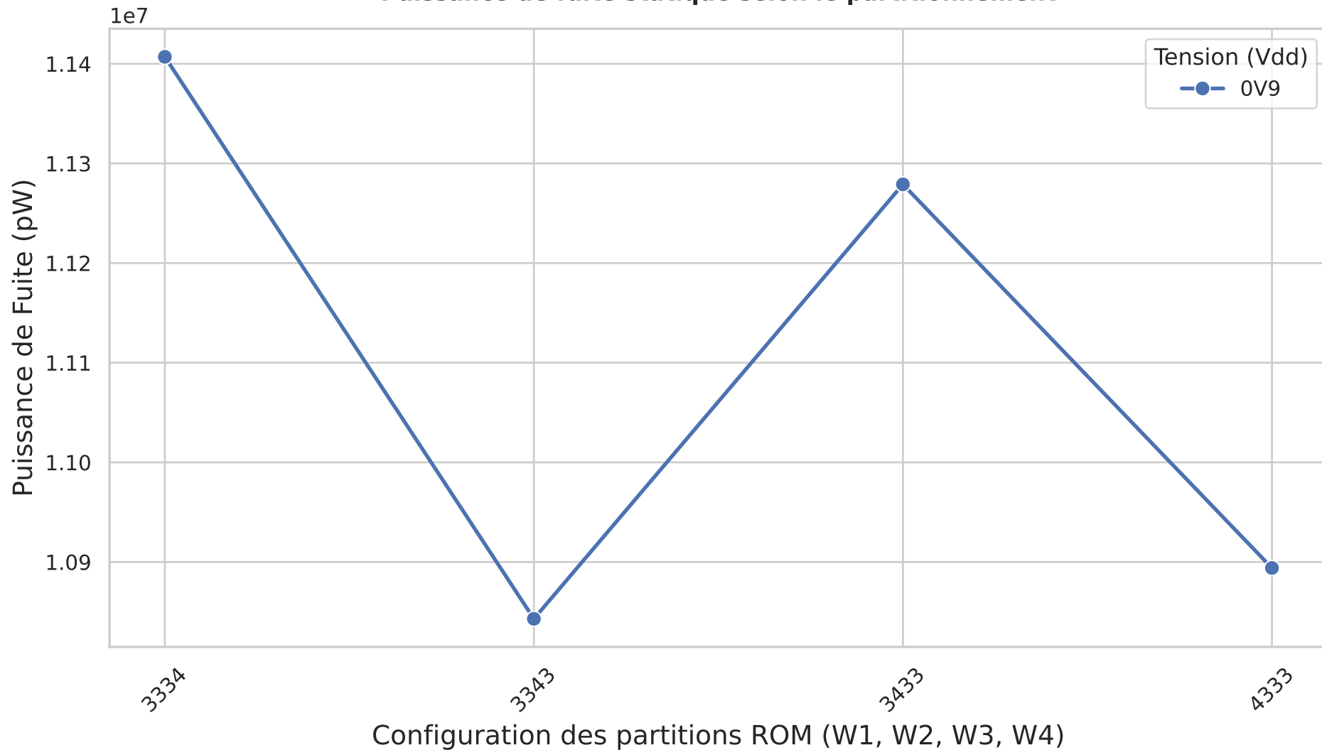
Puissance de fuite statique selon le partitionnement
