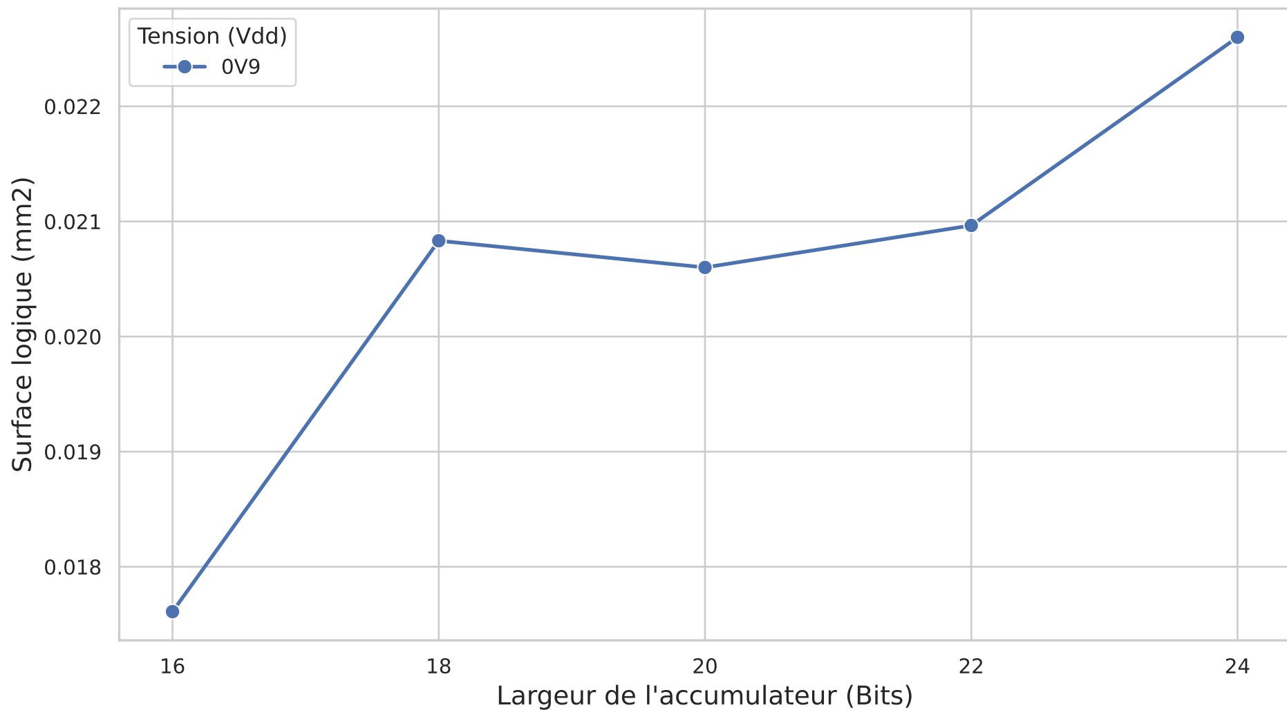
Empreinte silicium en fonction de la resolution
