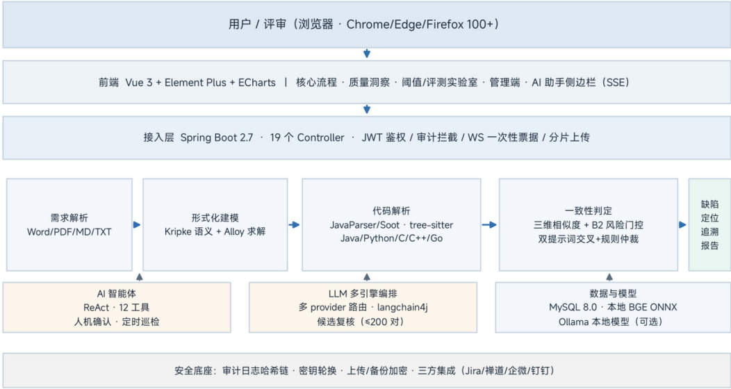
圖 1 系統總體架構
