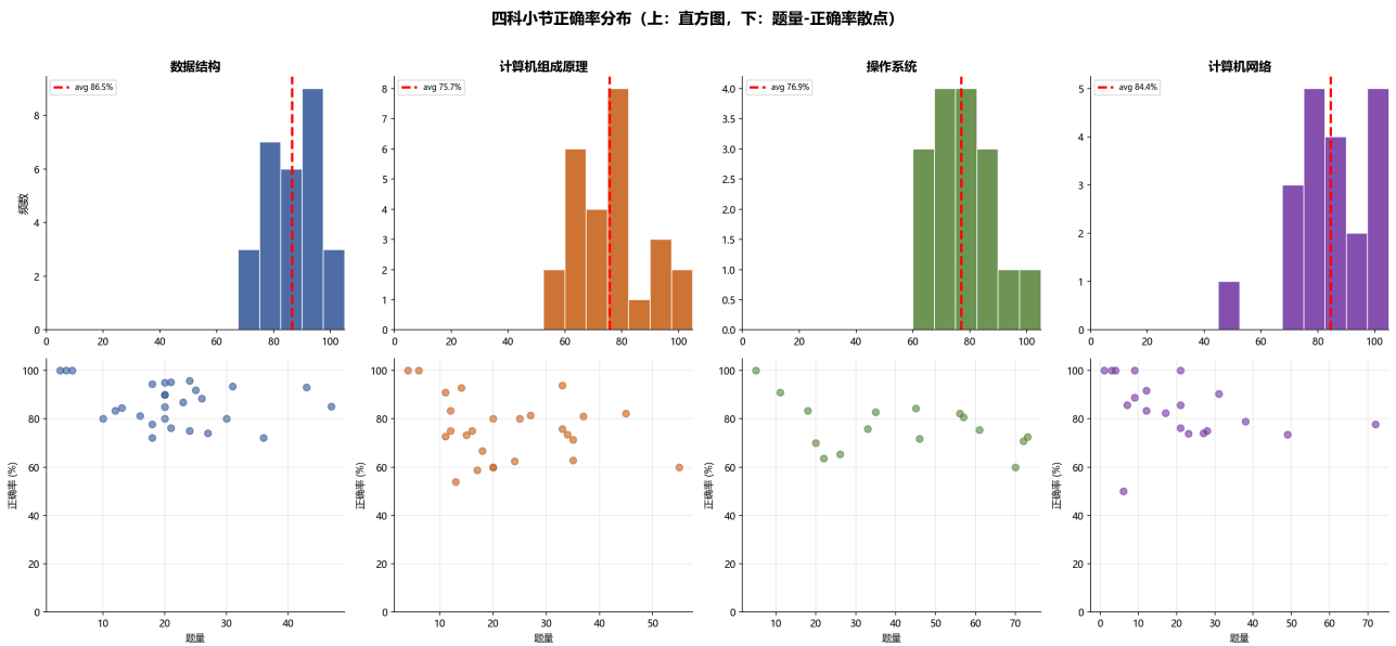
图 8: 上: 正确率直方图, 下: 题量-正确率散点图
