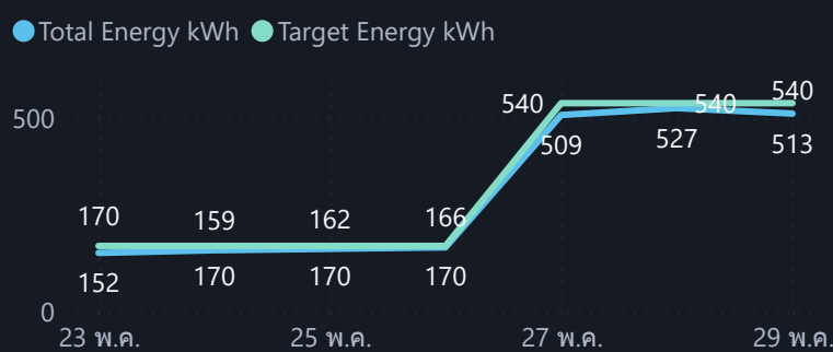
Daily Actual vs Target Energy
