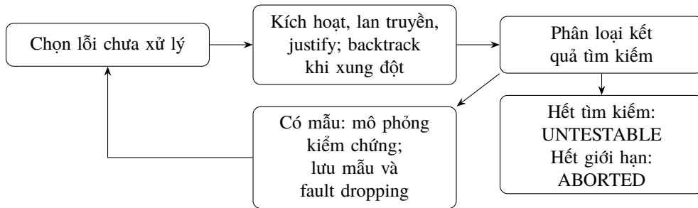
Hình 2.1: Luồng ATPG tất định và kiểm chứng mẫu.
