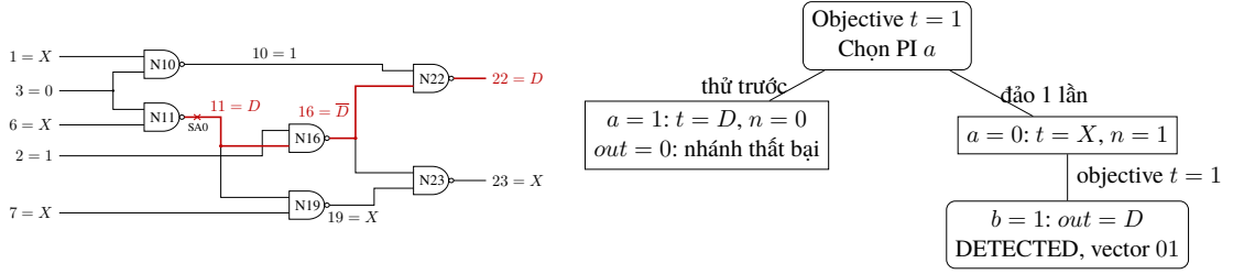
Hình 4.1: Trái: c17 ở trạng thái cuối. Phải: cây quyết định mạch phụ, thử a = 1 rồi đảo a = 0 .
