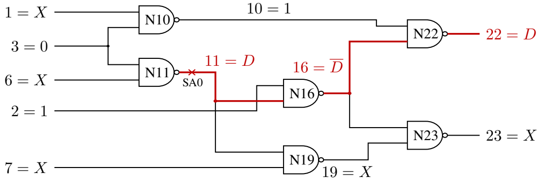
Hình 3.2: Mạch c17 với cube sau tổng quát hóa, 6 = X ; đường quan sát 11 = D \rightarrow 16 = D' \rightarrow 22 = D .
