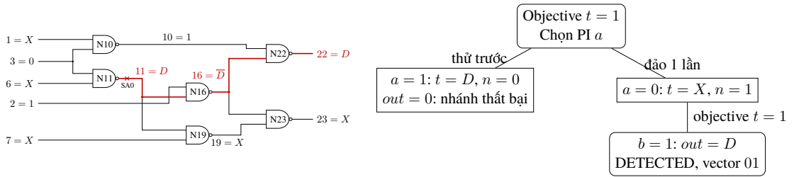
Hình 4.1: Trái: c17 ở trạng thái cuối (hình P2 nếu có; dự phòng P3: mọi khối là NAND). Phải: cây quyết định mạch phụ, thử a = 1 rồi đảo a = 0 .
