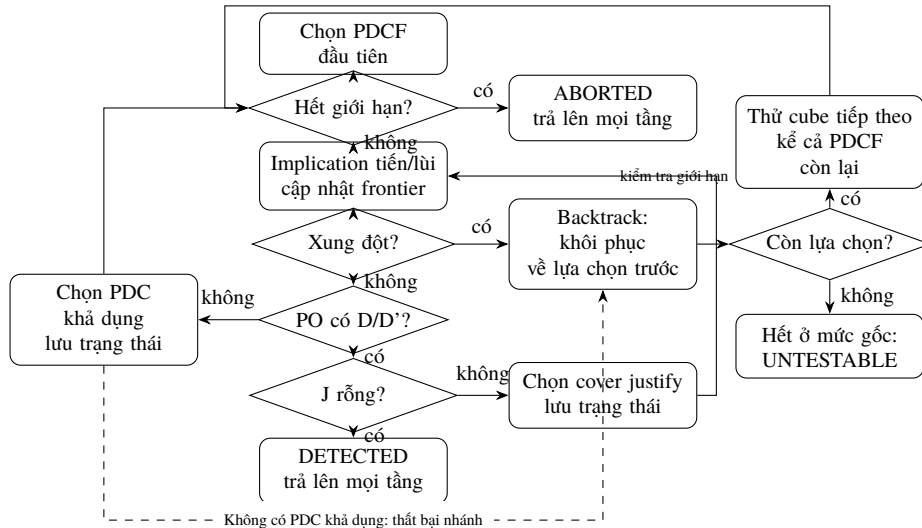
Hình 3.1: Luồng D-algorithm; khôi phục cả gán net và frontier khi quay lui.
