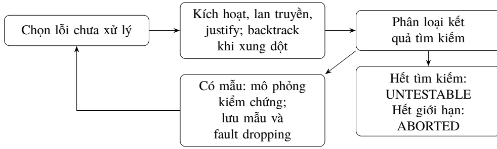
Hình 2.1: Luồng ATPG tắt định và kiểm chứng mẫu.
