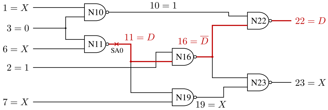
Hình 3.2: Hình c17 do P2 cung cấp: cube sau tổng quát hóa, 6 = X ; đường quan sát 11 = D \rightarrow 16 = D' \rightarrow 22 = D .
