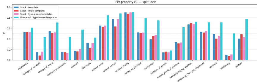
Figure 7: Per-property F1
