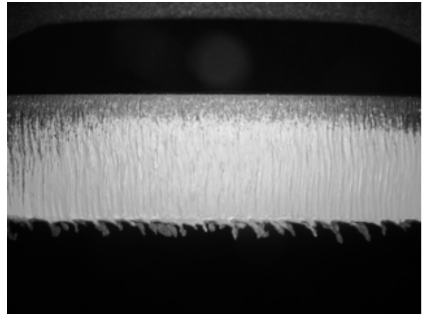
Abb. 13: Handcanner Bild für die Gratschätzung (Edelstahl)
