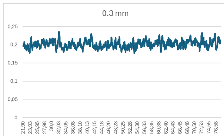
Abb. 17: Beispielhafter Verlauf der Rauheitskennzahl R_a entlang einer Schnittkante im ersten Abschnitt mit der Breite 0,3 mm.
