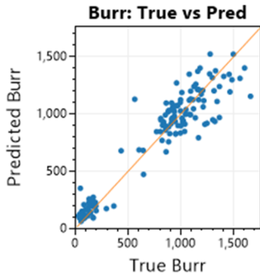
Abb. 9: Vergleich zwischen vorhergesagten und tatsächlichen Werten für den Grat (Burr).
