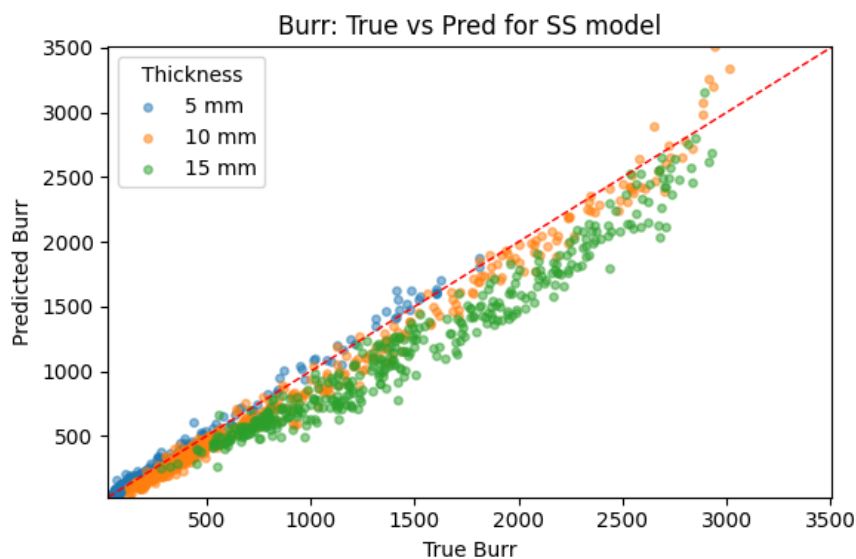
Abb. 21: Burr: wahre gegen vorhergesagte Werte für das SS-Modell. Die Farben kennzeichnen 5 mm, 10 mm und 15 mm. Die gestrichelte Diagonale markiert y=x .
