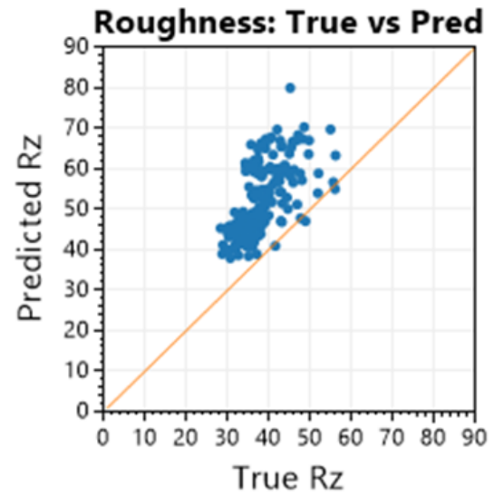
Abb. 10: Vergleich zwischen vorhergesagten und tatsächlichen Werten für die Rauheit (Roughness).
