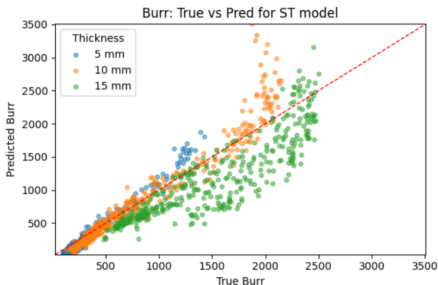
Abb. 20: Burr: wahre gegen vorhergesagte Werte für das ST-Modell. Die Farben kennzeichnen 5 mm, 10 mm und 15 mm. Die gestrichelte Diagonale markiert y=x .
