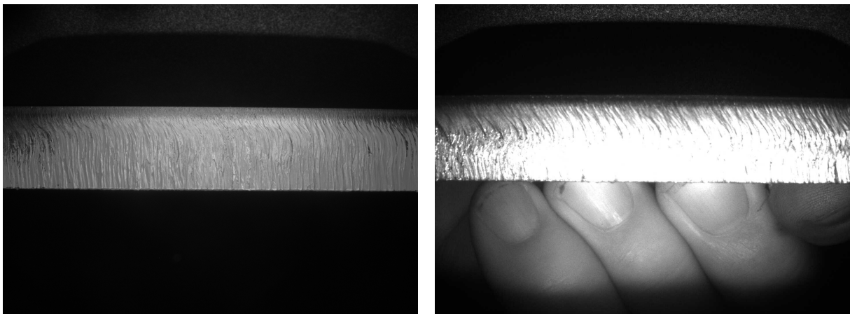
Abb. 3: Beispiele zur Plausibilitätsprüfung durch „Iron-hunter“: links eine gültige Aufnahme der Schnittkante, rechts eine Fehlaufnahme mit verdeckender Hand, die verworfen wird.
