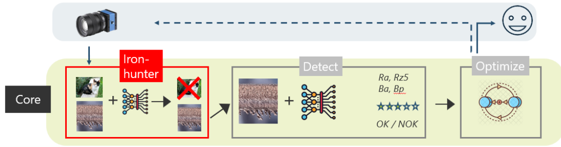
Abb. 4: Prozesskette des Cutting Assistant.
