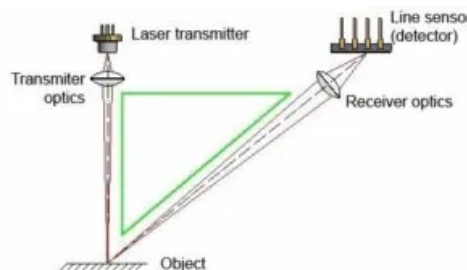
Abb. 5: Lasertriangulation zur Profilaufnahme. (Sensor Instruments GmbH 2023)
