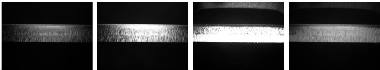
Abb. 11: Dunkle Belichtung für die Rauheitsschätzung (i, erstes Bild links), zwei helle Belichtungen für die Gratschätzung (ii, mittlere Bilder) und das daraus generierte HDR-Bild (rechts).
