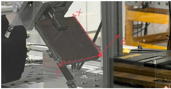
Abb. 6: Messaufbau und Beispielpunktwolke der Schnittkante für den Gratverlauf.
