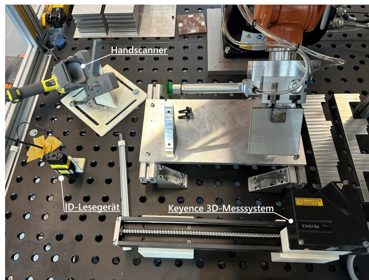
Abb. 10: Handscanner (1), ID-Lesegerät (2), Keyence 3D-Messsystem (3) in der Messzelle
