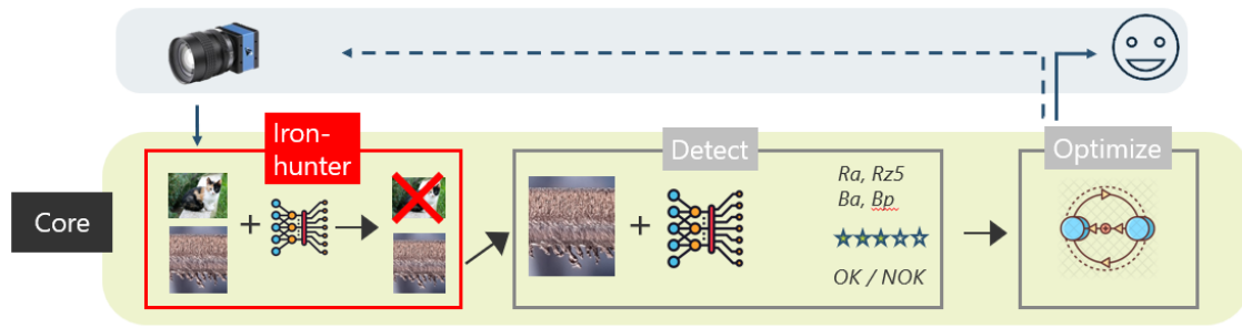
Abb. 7: Prozesskette des Cutting Assistant.
