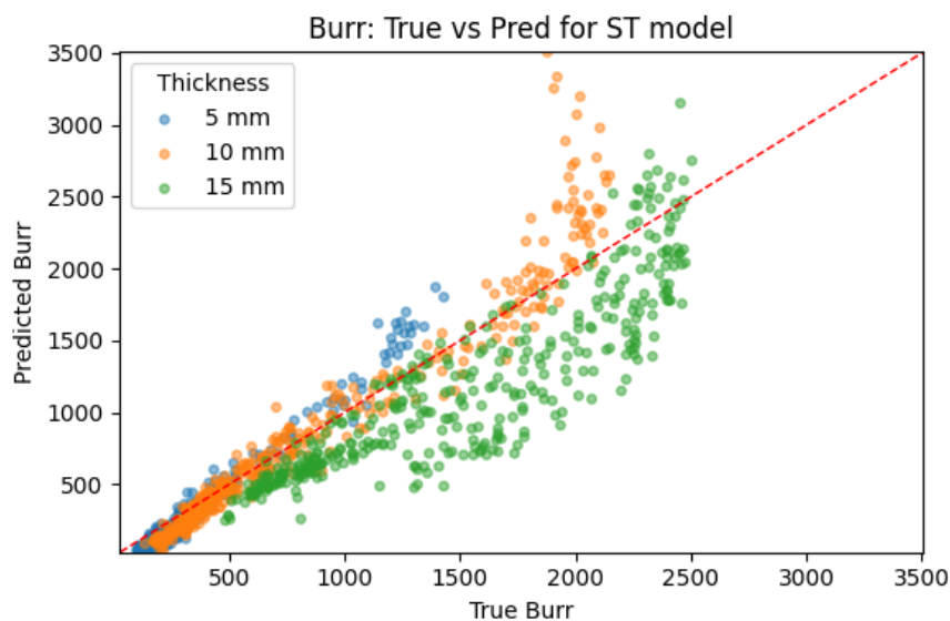
Abb. 23: Burr: wahre gegen vorhergesagte Werte für das ST-Modell. Die Farben kennzeichnen 5 mm, 10 mm und 15 mm. Die gestrichelte Diagonale markiert y=x .
