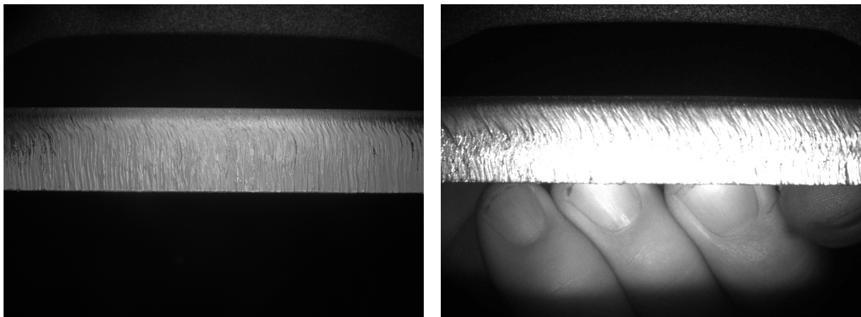
Abb. 6: Beispiele zur Plausibilitätsprüfung durch „Iron-hunter“: links eine gültige Aufnahme der Schnittkante, rechts eine Fehlaufnahme mit verdeckender Hand, die verworfen wird.
