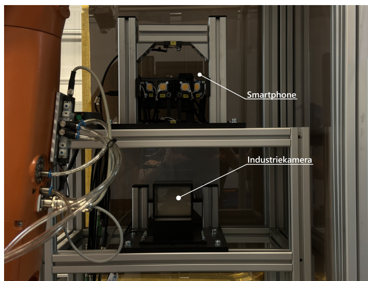
Abb. 11: Smartphone (4) und Industriekamera (5) in der Messzelle
