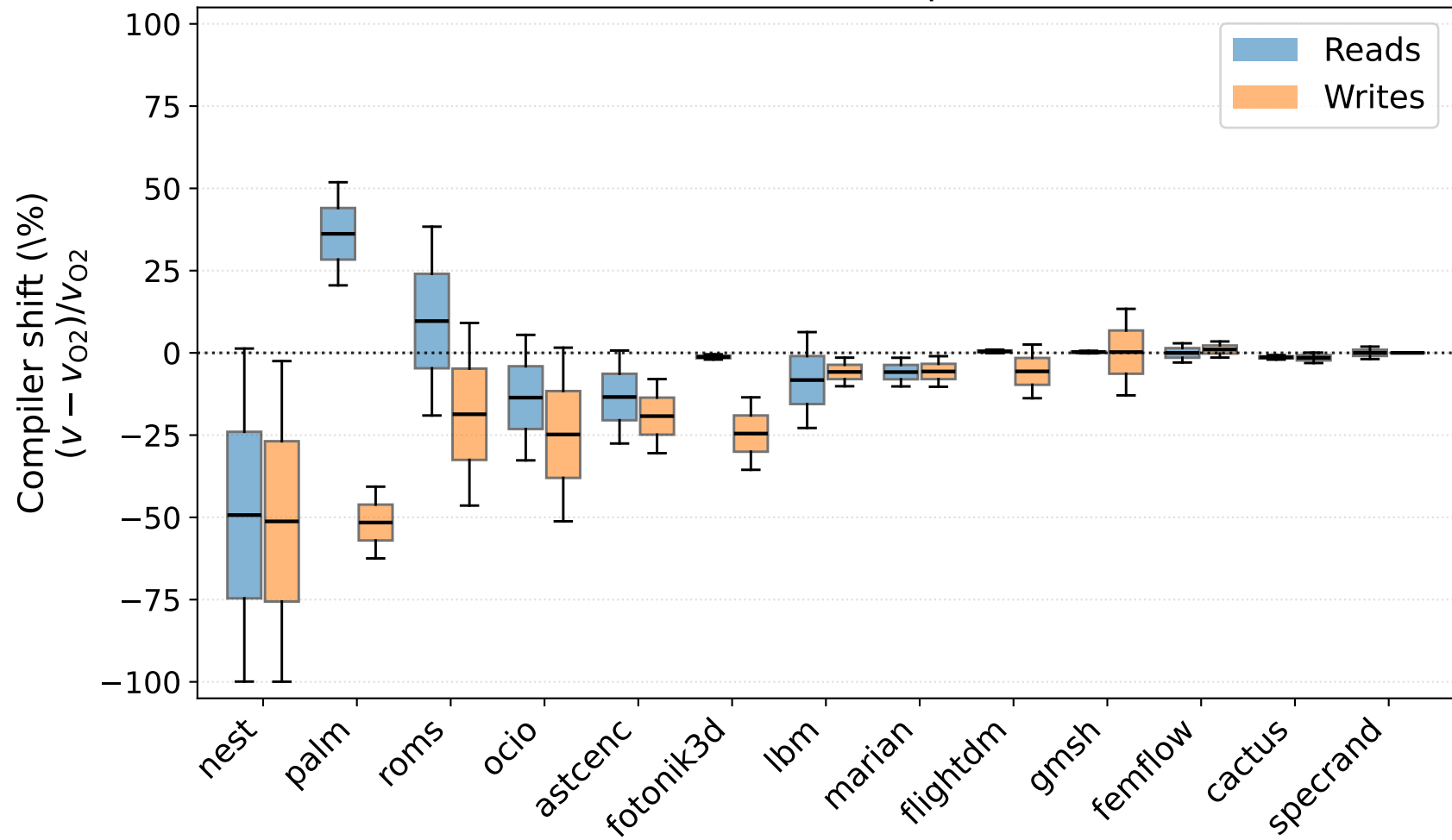
SPEC CPU2026 fprate
