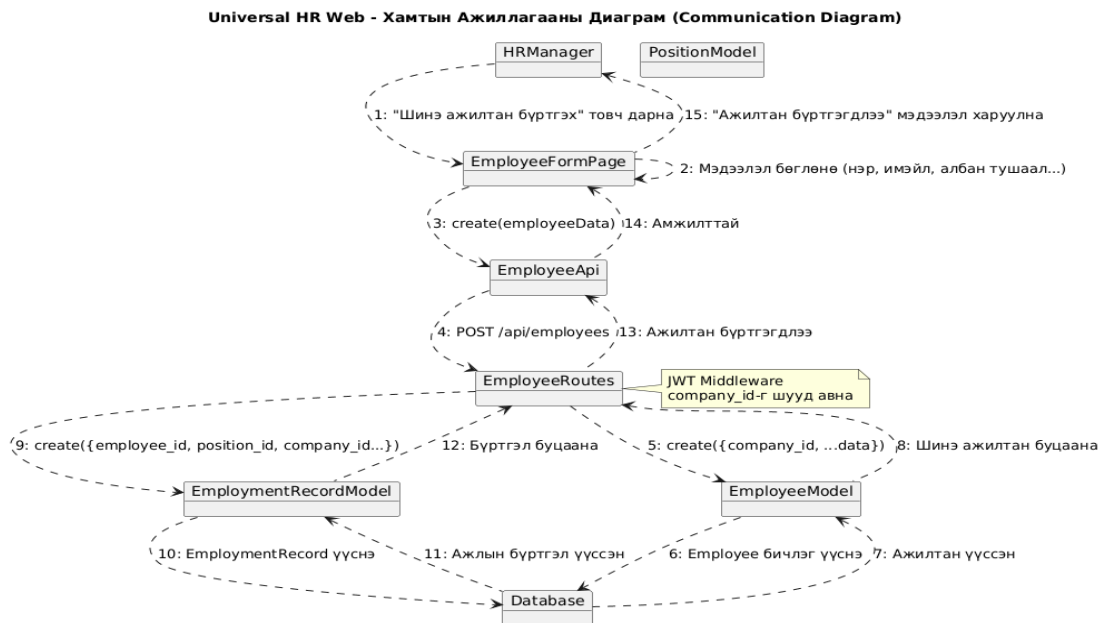
Зураг 14 Collaboration диаграмм
