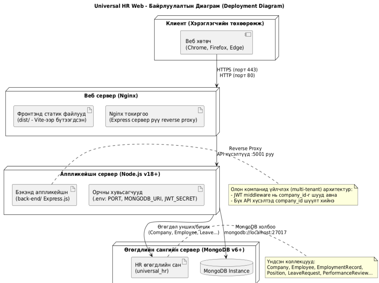
Зураг 16 Deployment диаграмм
