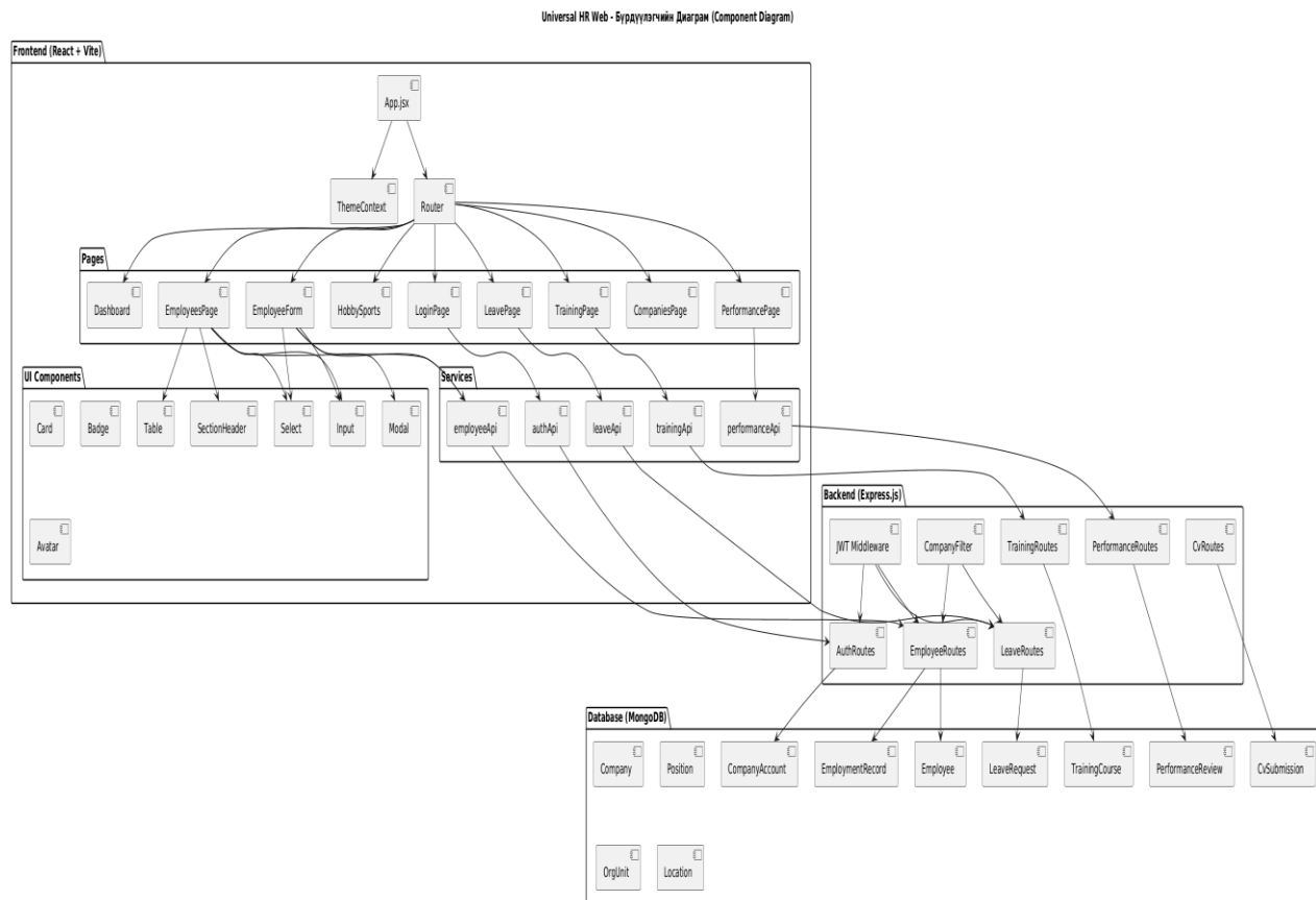
Зураг 15 Component диаграмм
