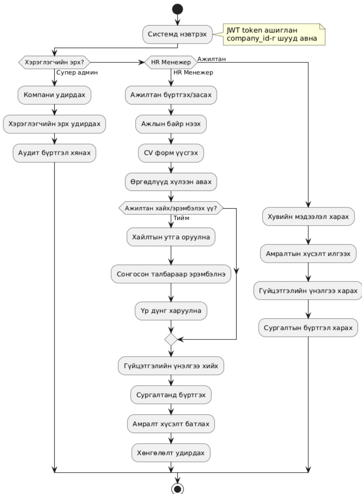
Universal HR Web - Үйл Ажиллагааны Диаграм (Activity Diagram)
