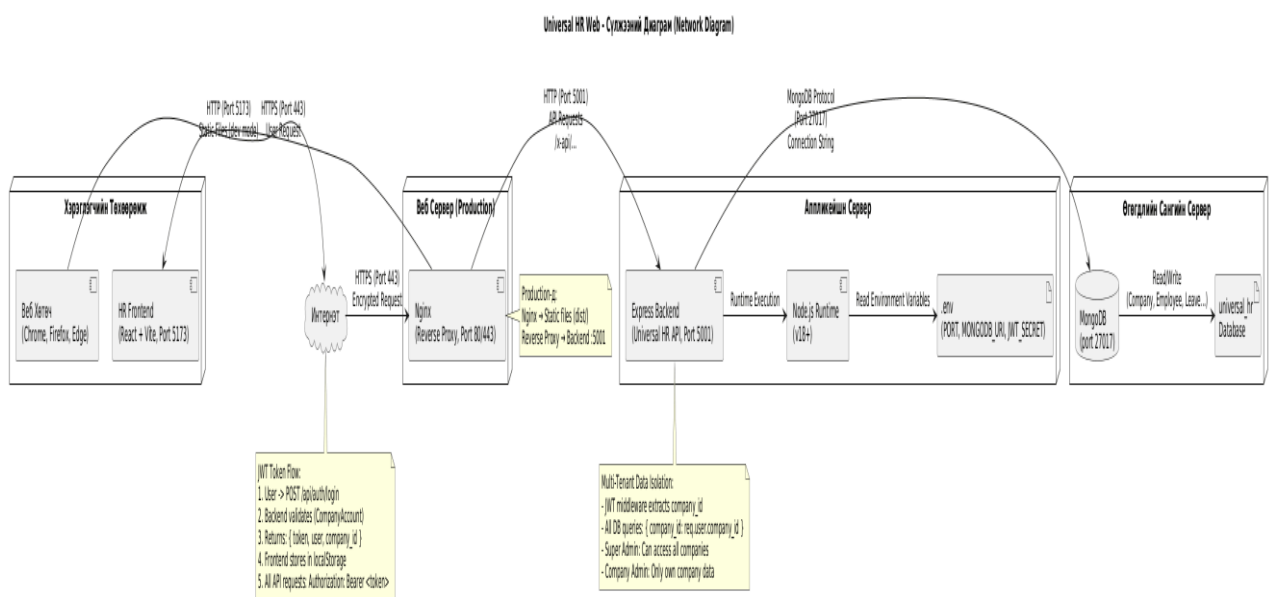
Зураг 17 Network диаграмм
