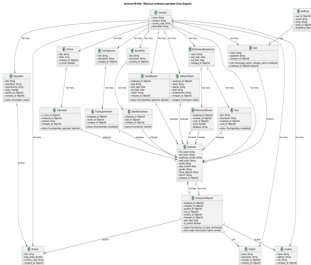
Зураг 8 Объектын холбоосон диаграмм
