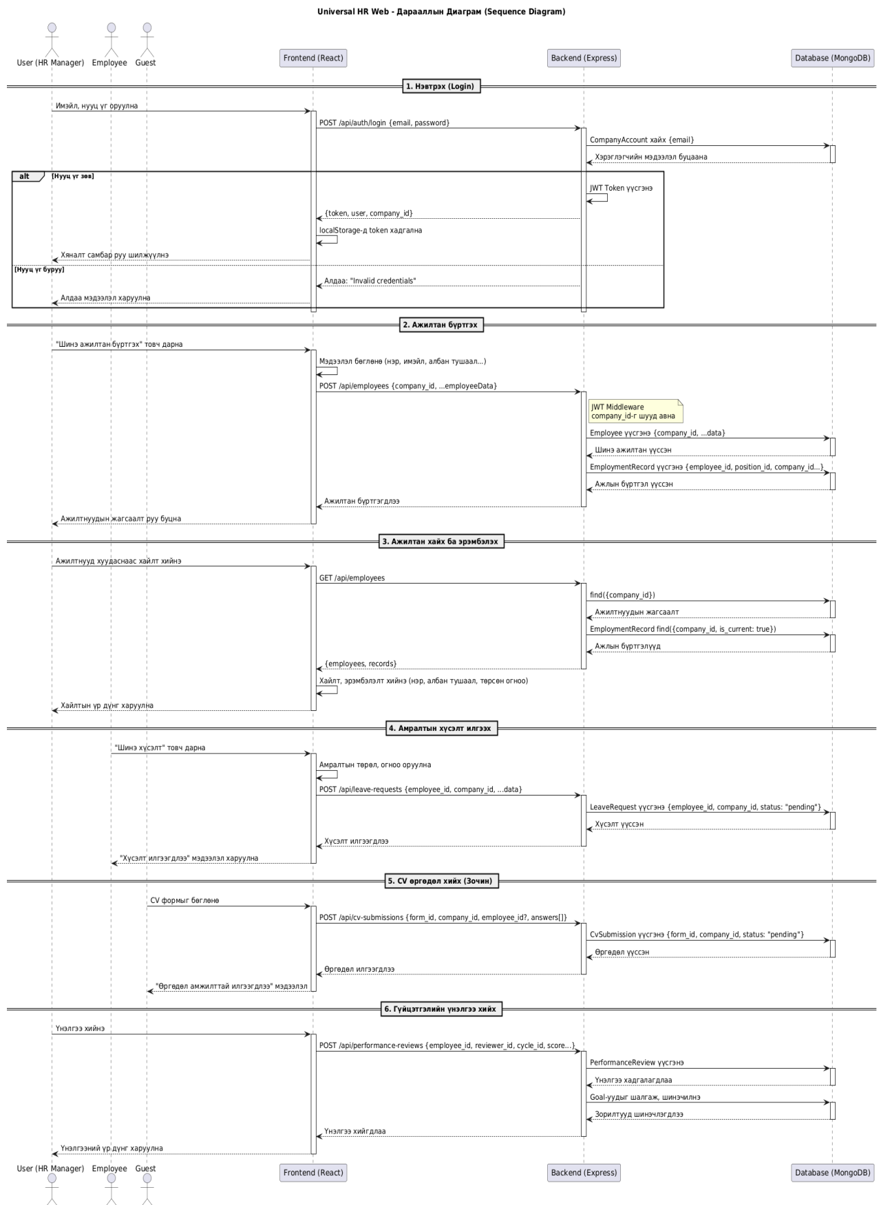
Зураг 11 Sequence диаграмм
