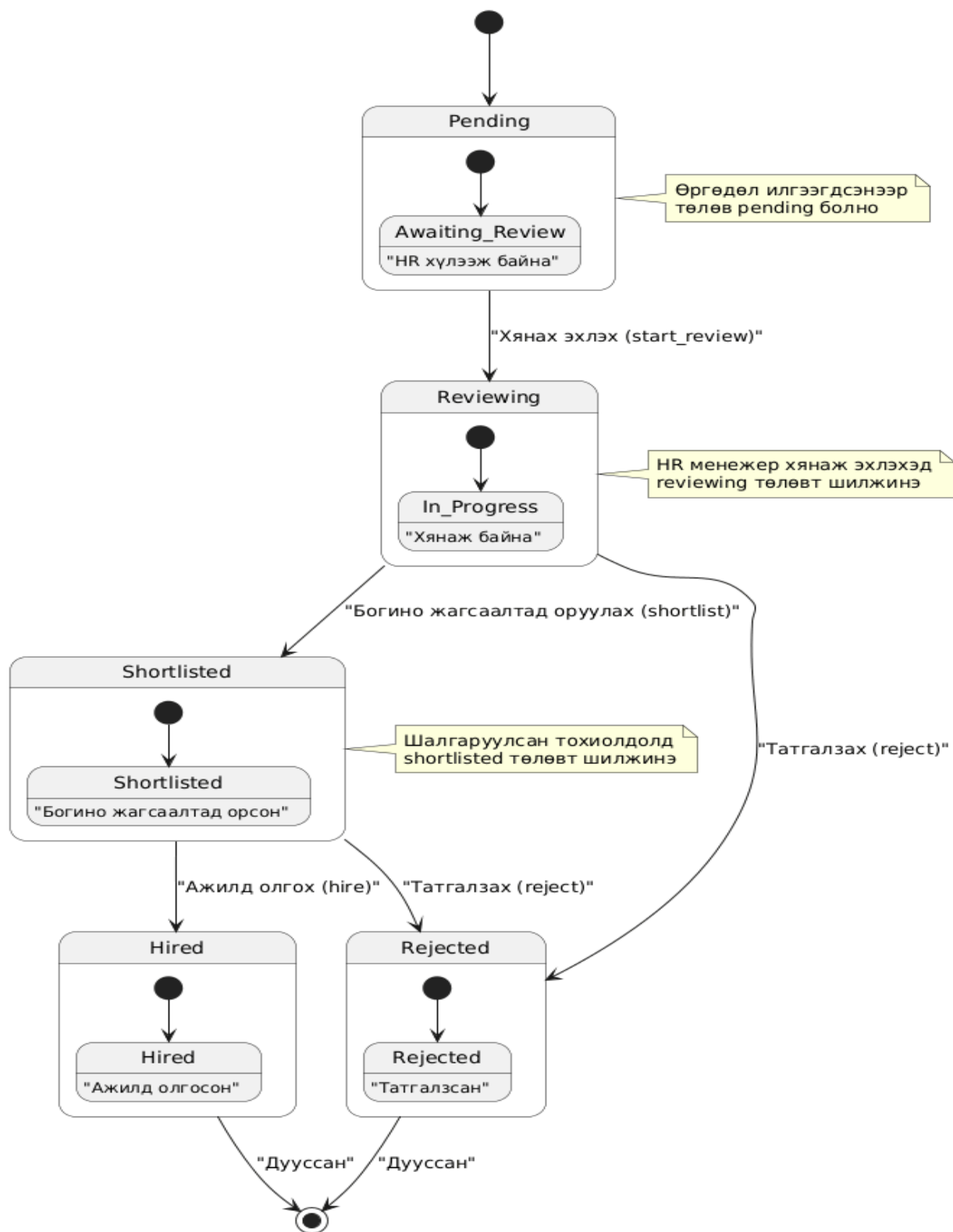
CvSubmission - Төлвийн Диаграм (State Chart Diagram)
