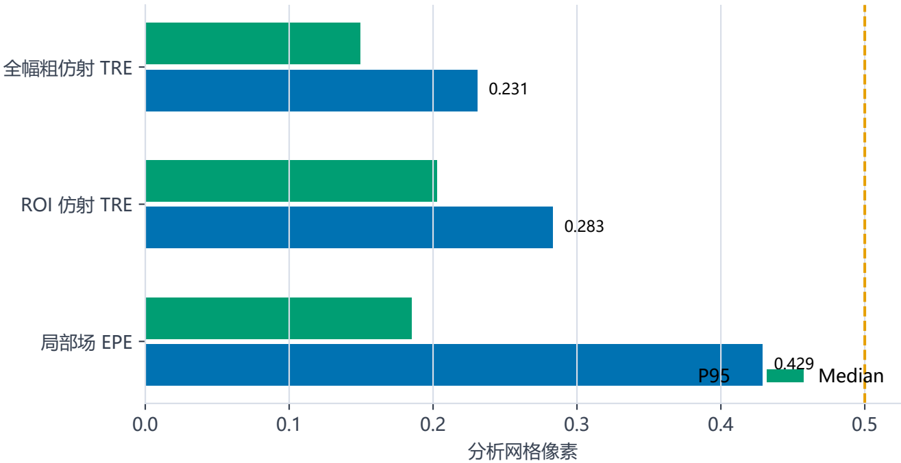
受控合成真值：组件级亚像素证据
