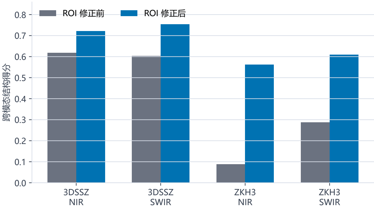
真实 ROI：配准结构得分提升
