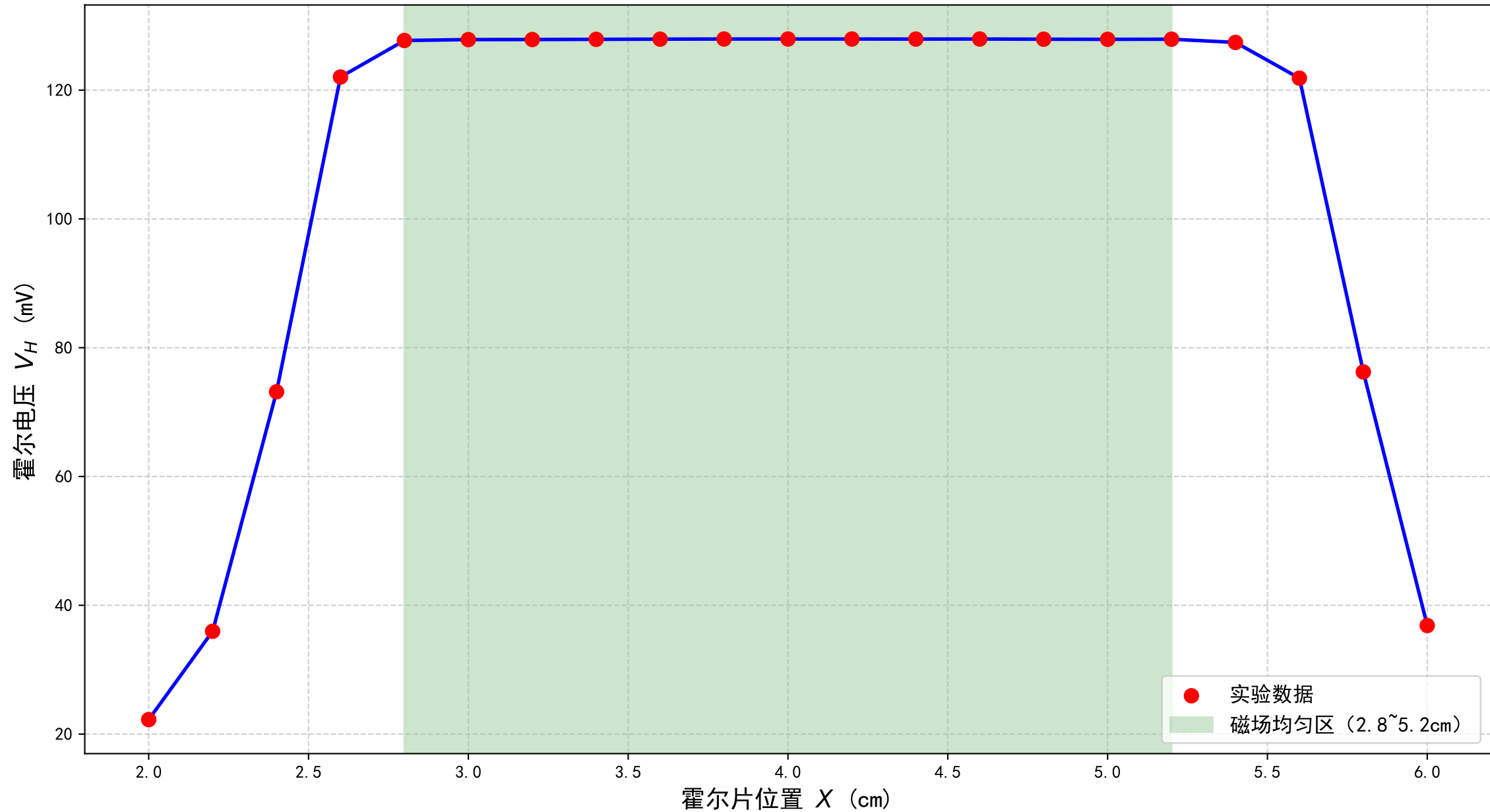
电磁铁气隙磁场分布： X - V_H 关系曲线
