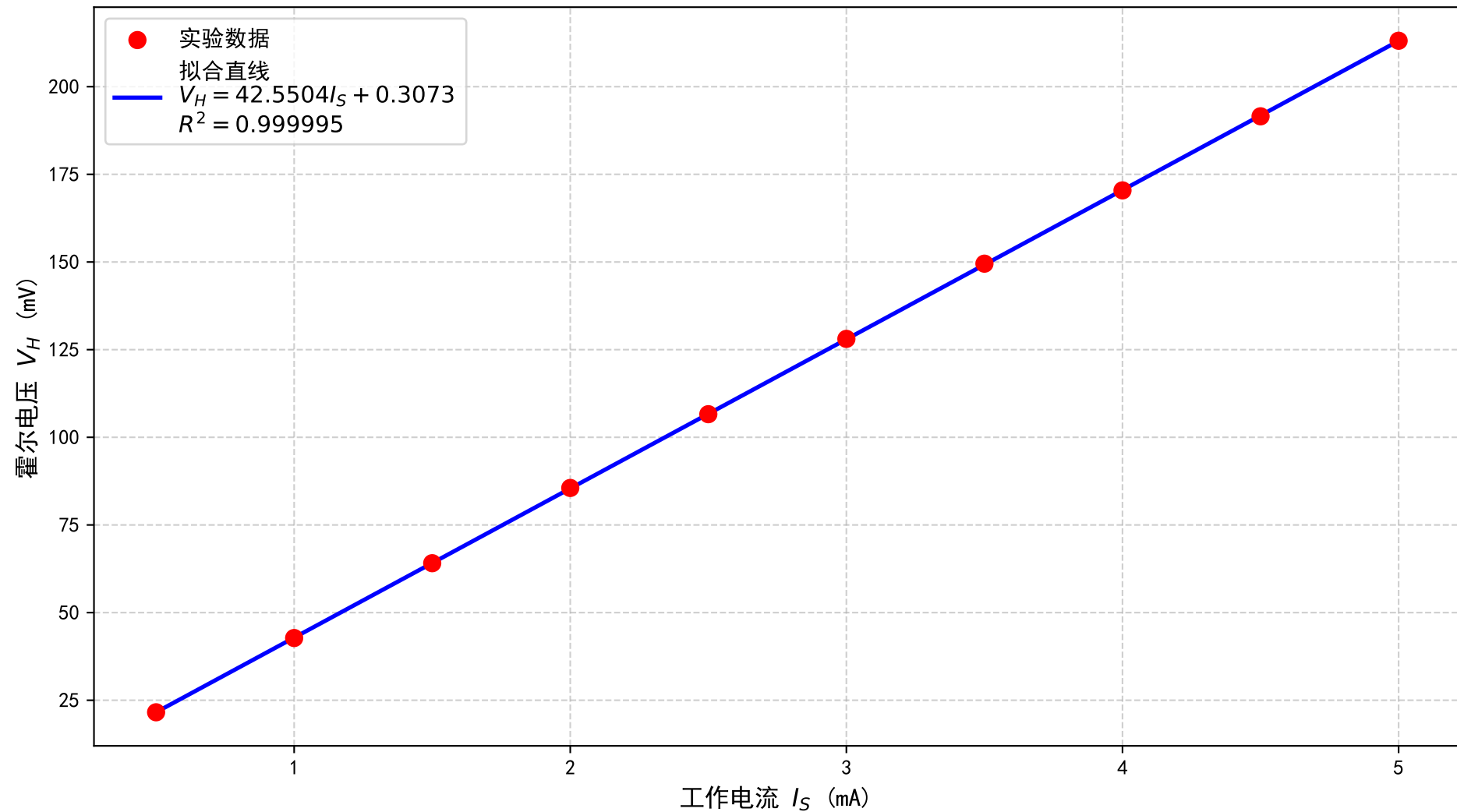
霍尔效应: V_H - I_S 线性关系拟合
