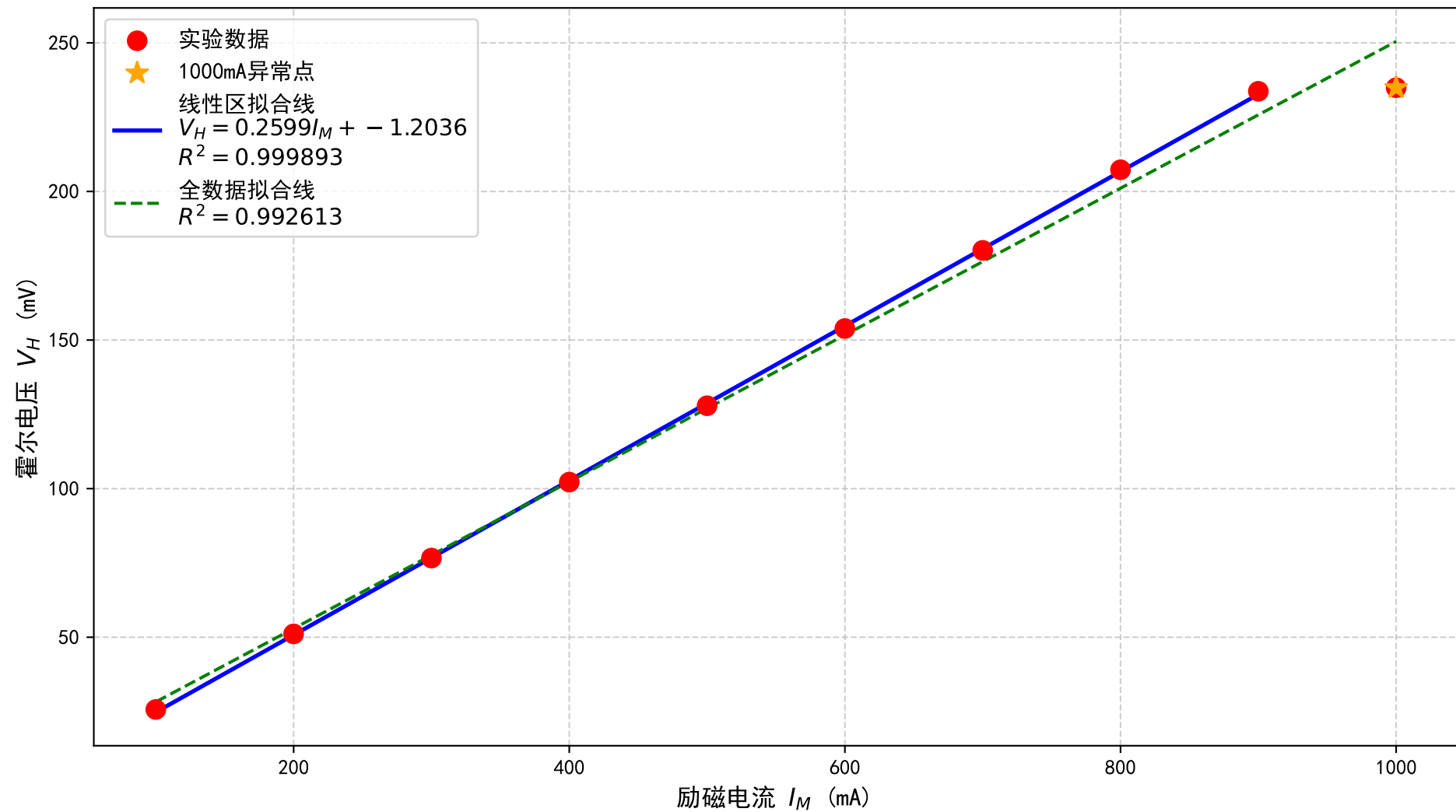
霍尔效应： I_M - V_H 关系拟合与线性范围验证
