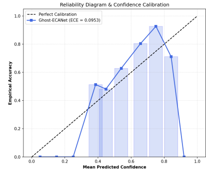
(c) Kalibrasyon Eğrisi (ECE: 0.095)
