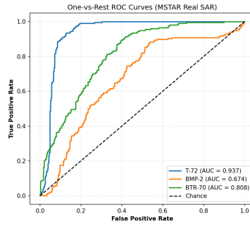
(b) ROC Eğrileri (T-72: 0.937)
