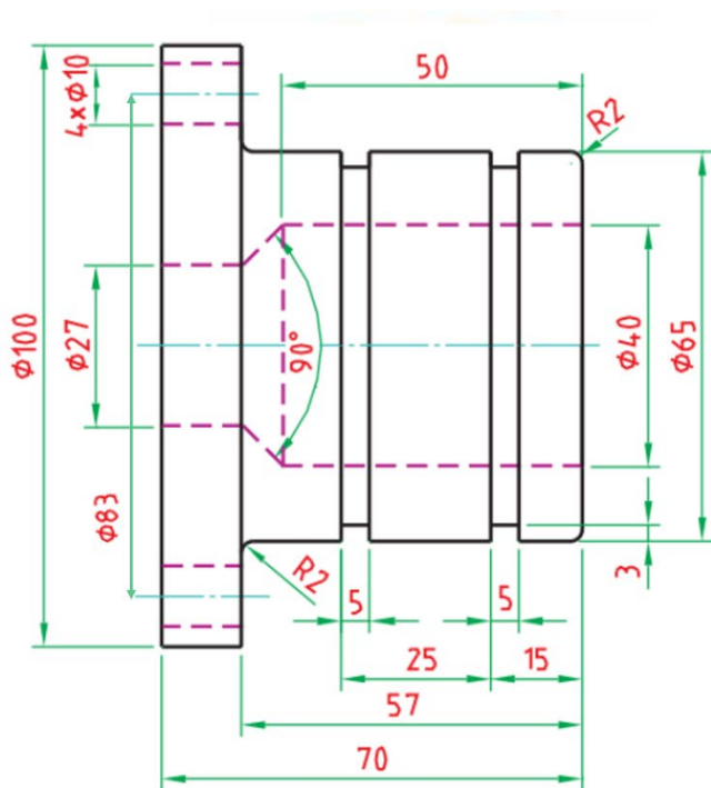
前視圖
