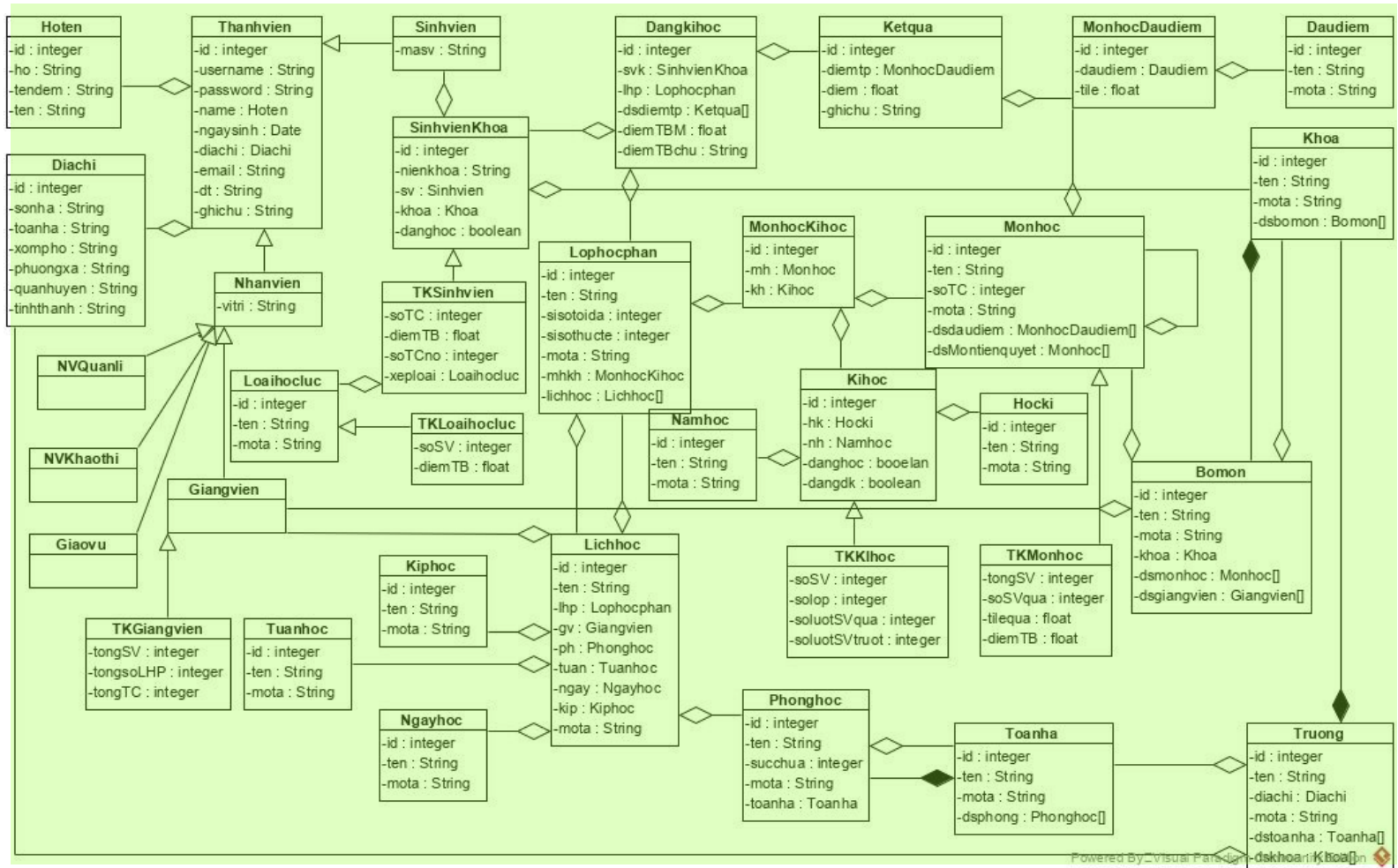
Hình 4.1: Biểu đồ thiết kế lớp thực thể 3
