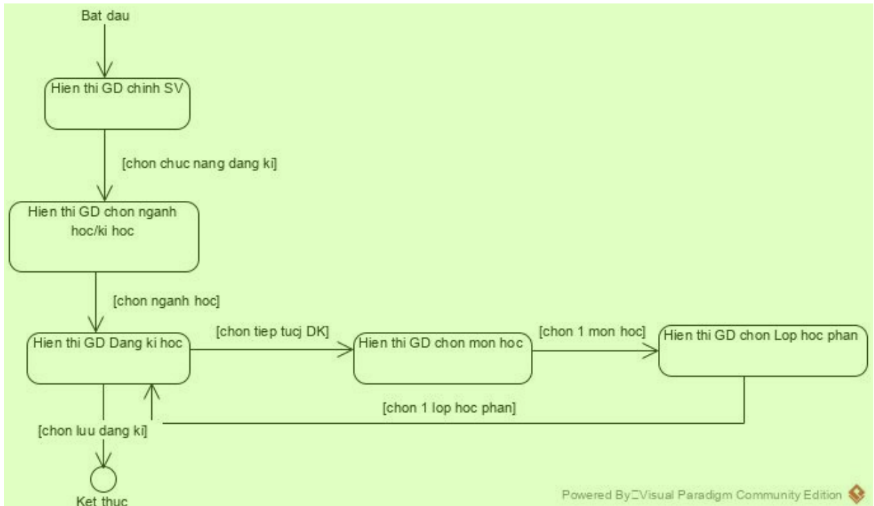
Hình 3.9: Biểu đồ chuyển trạng thái của modul đăng kí học 4
