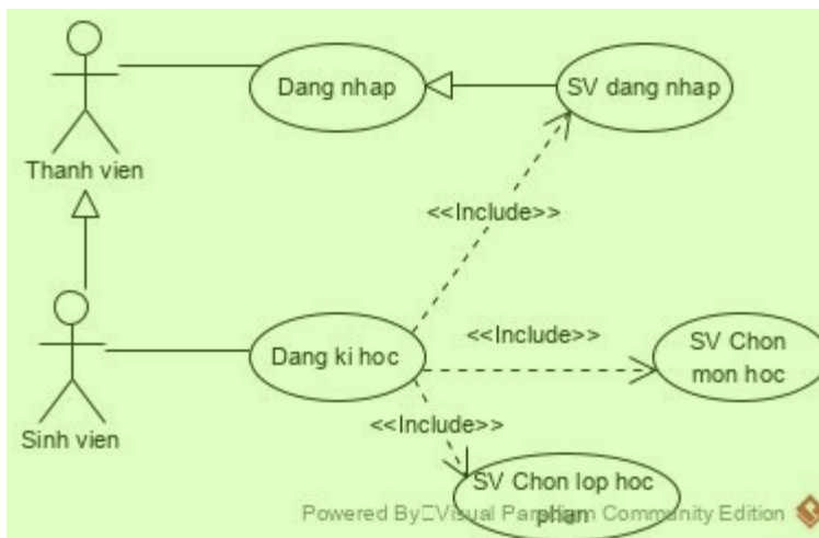
Hình 3.2: Biểu đồ use case
