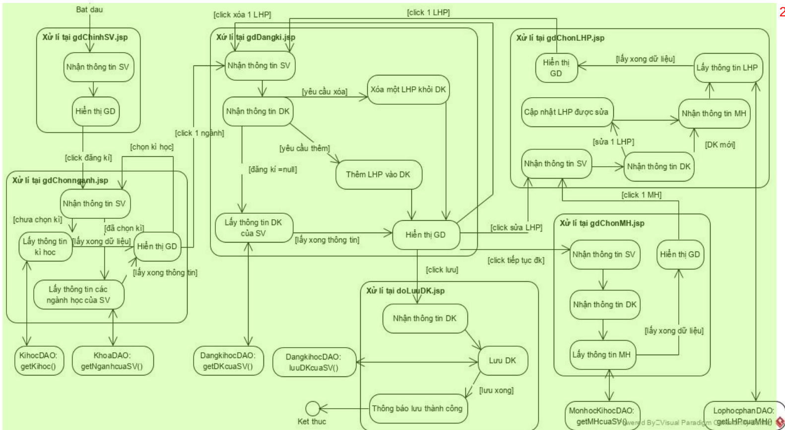
Hình 4.9: Biểu đồ thiết kế hoạt động modul đăng kí học 3
