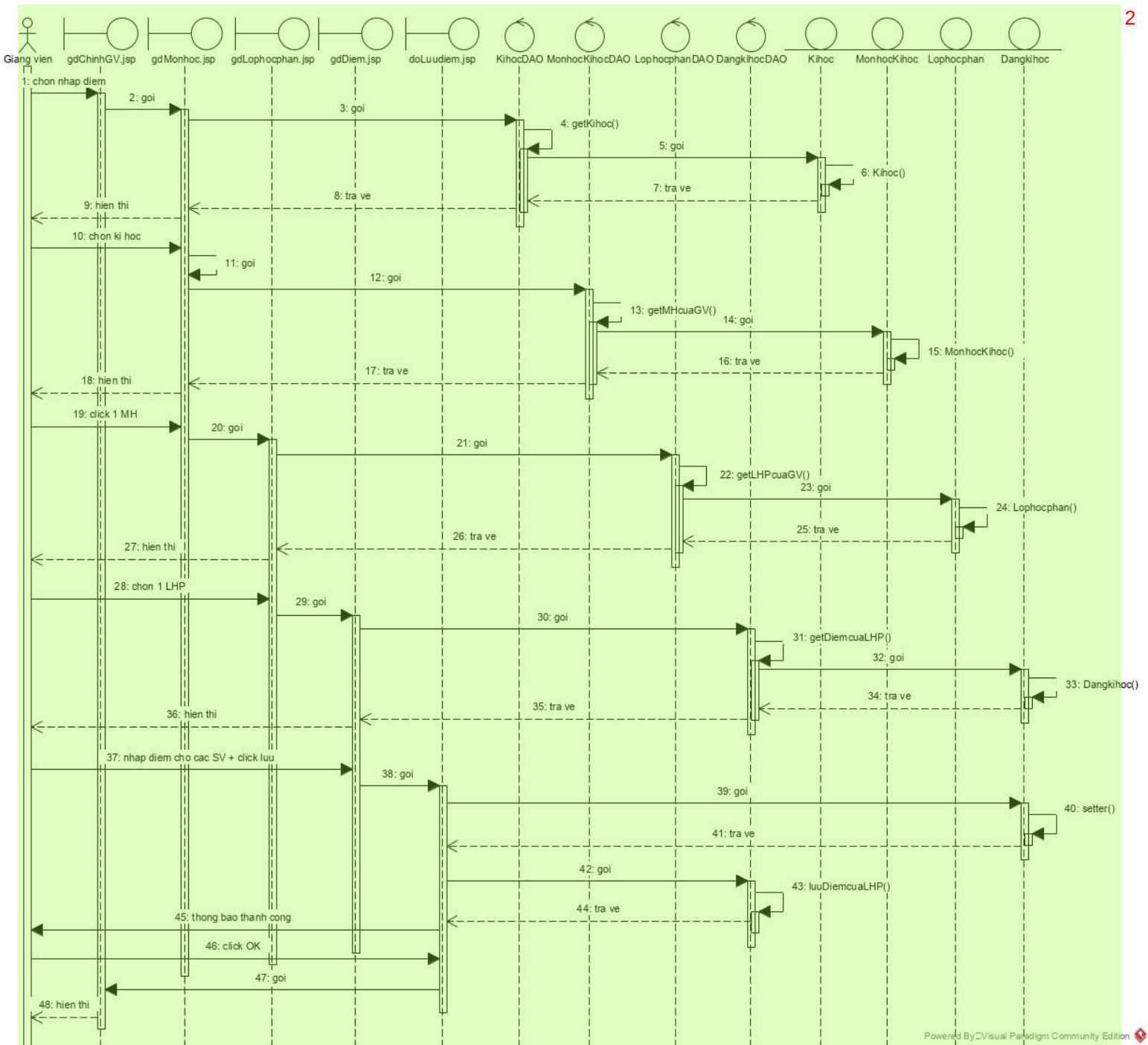
Hình 4.12: Biểu đồ tuần tự thiết kế modul nhập điểm 3
