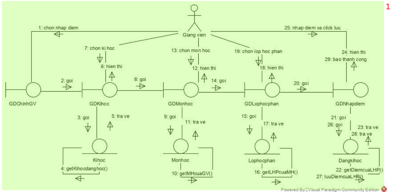
Hình 3.12: Biểu đồ giao tiếp của modul nhập điểm 2
