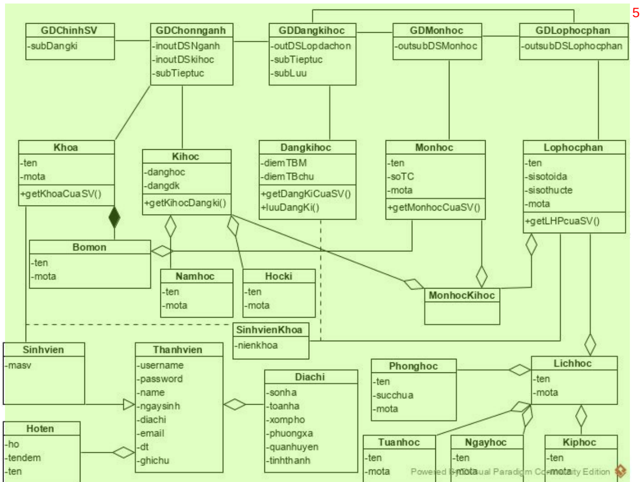
Hình 3.6: Biểu đồ lớp phân tích modul đăng kí học 6
