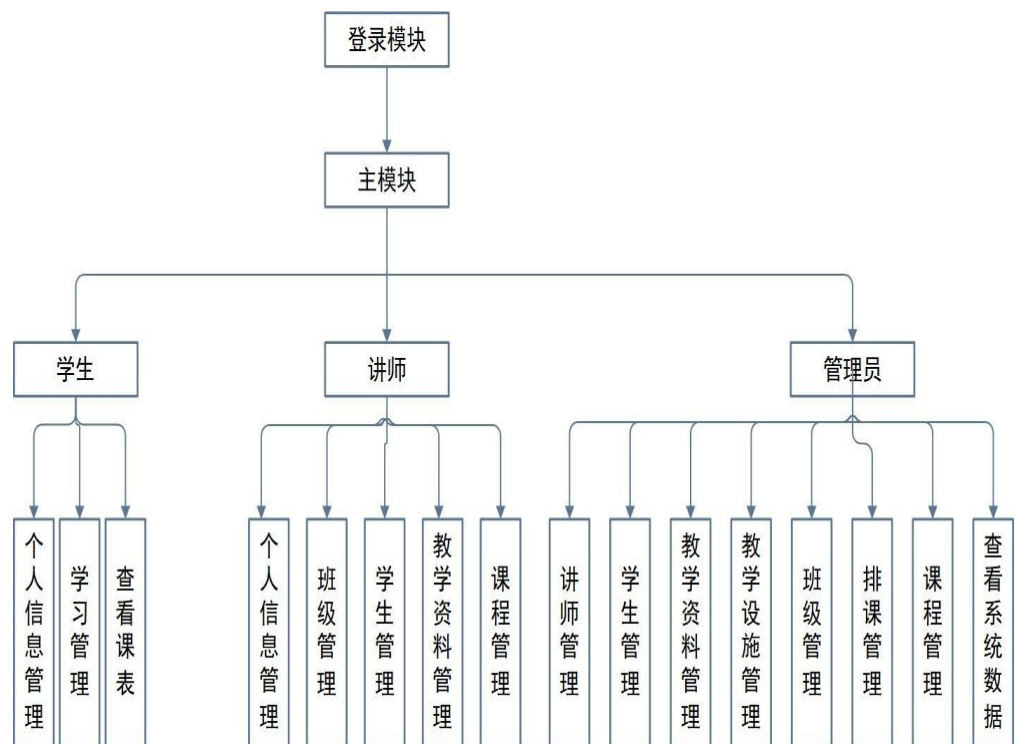
图 5 中小学智能排课管理系统功能框图
