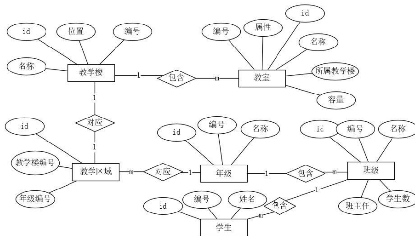
图 4.3 教学楼、教室、教学区域、年级、班级与学生实体的 ER 图
