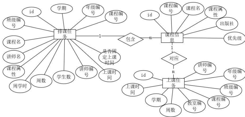
图 4.2 排课任务、课程信息与上课任务实体的 ER 图
