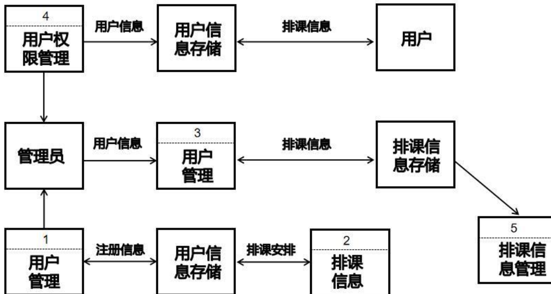
图 4.5 系统 0 层数据流图
