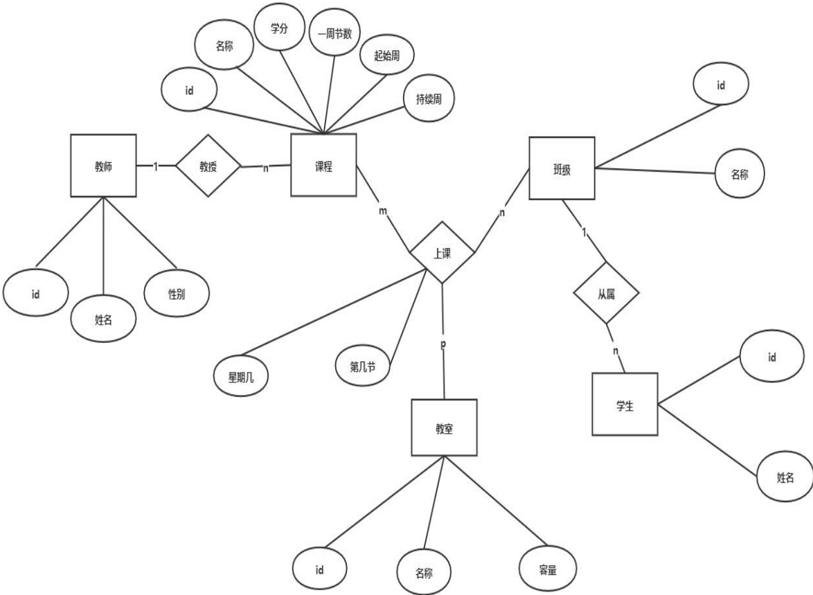
图 4.1 中学排课管理系统三个大实体间的 ER 图
