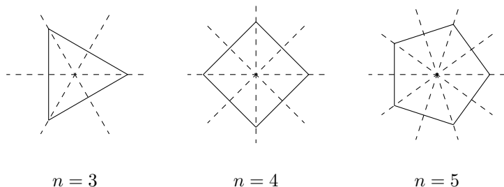
图 11-1: 二面体群包含的镜射
