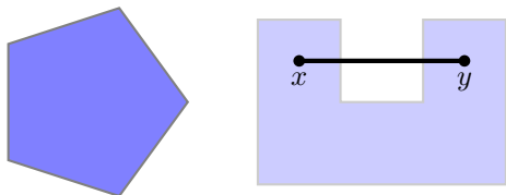
图 14-5: 凸与非凸子集
