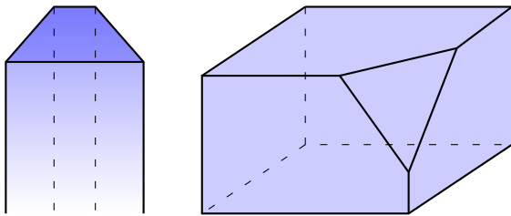
图 14-7: 多面体和多胞体
