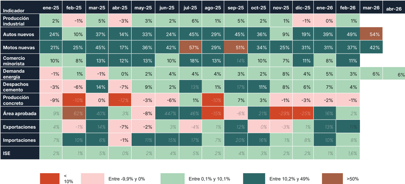
Figura 2. Mapa de calor de los principales indicadores líderes en Colombia.
