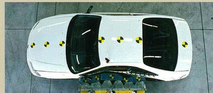
側面衝突実験(50km/h、写真は実験用の試作車です。)
