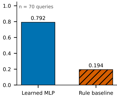
Held-out AUC
