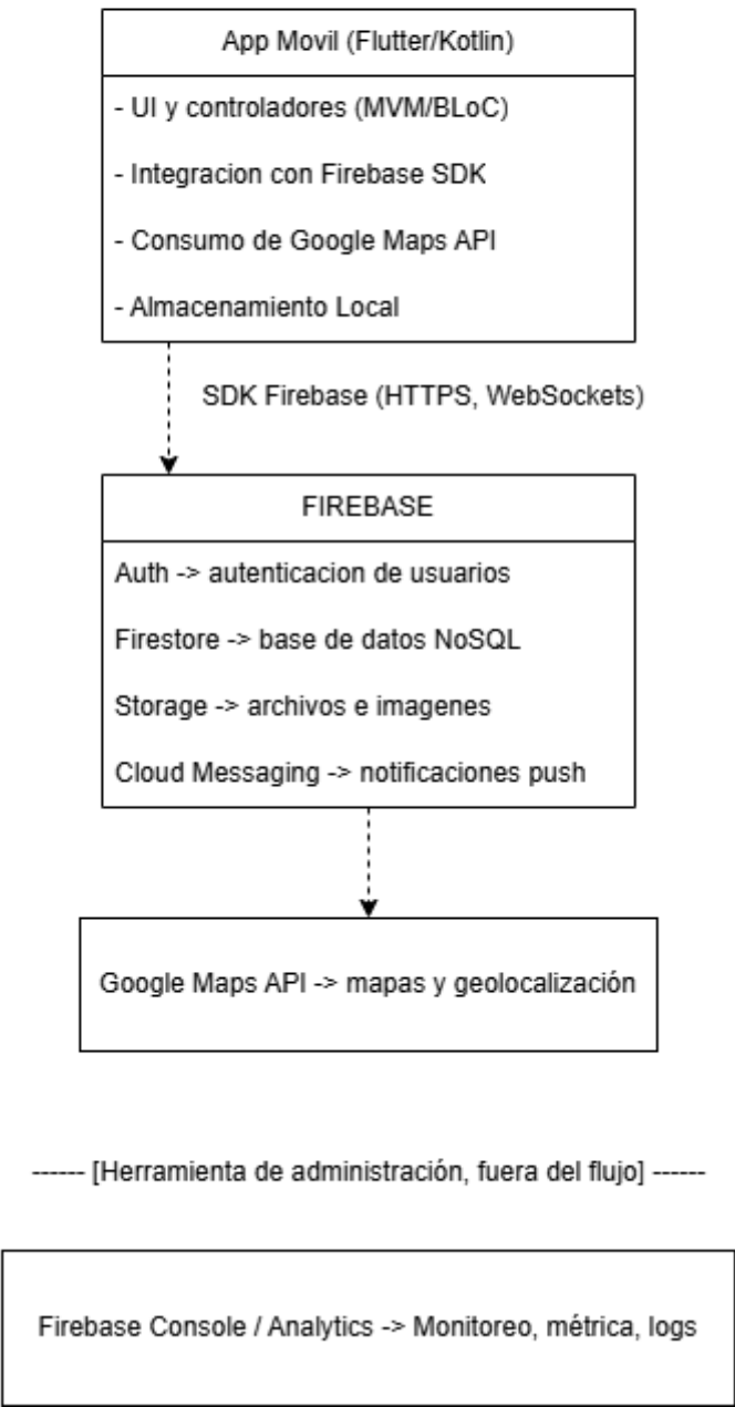
Ilustración 2: Diagrama C2 (Contenedores)
