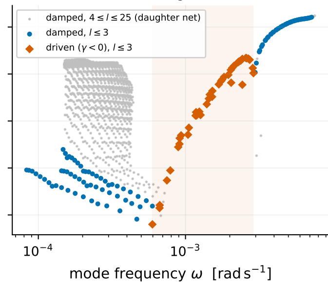
(d) all together
