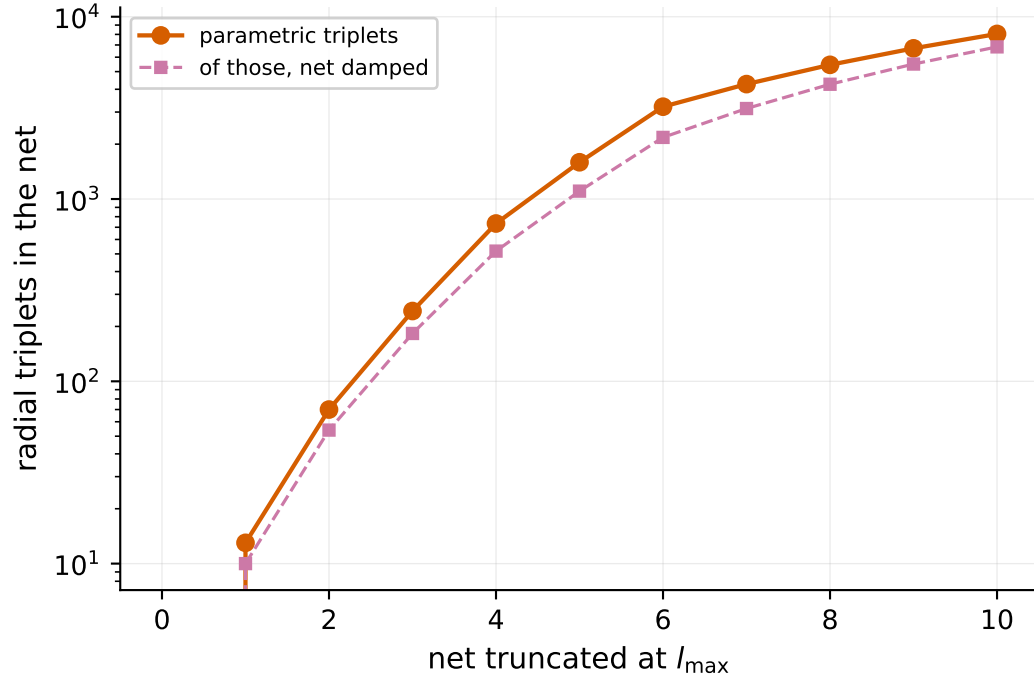
(d) supply of resonant triplets
