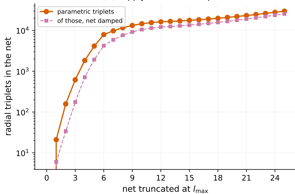
(d) supply of resonant triplets
