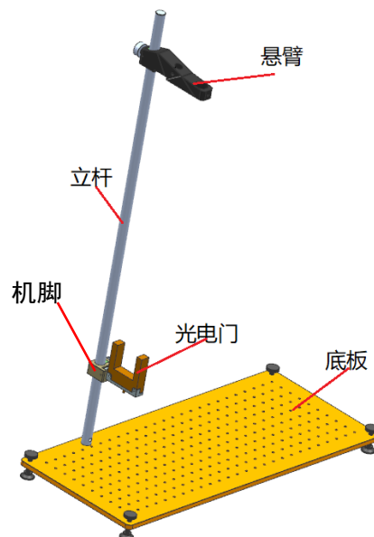
图 5 单摆实验装置图
