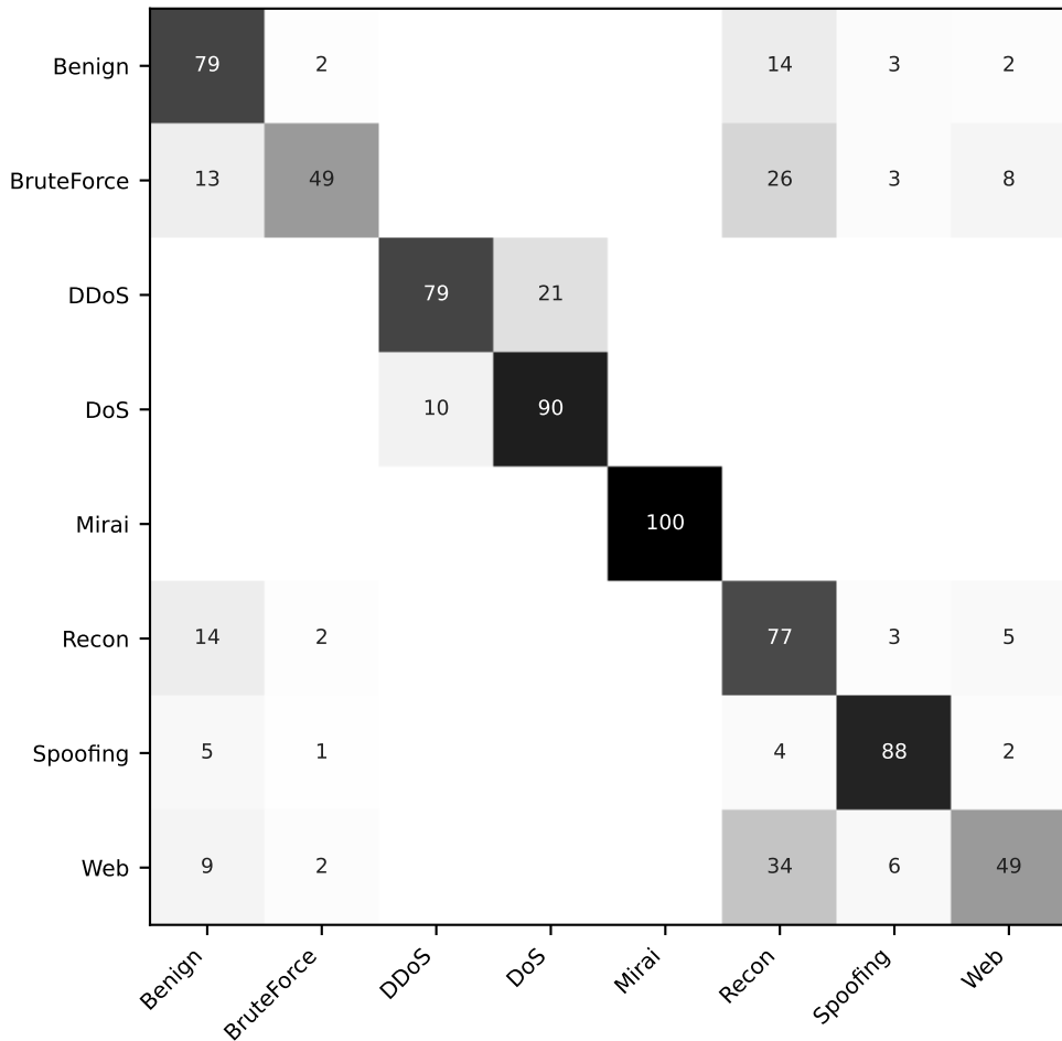
XGBoost — test aibē, atkūrimas kategorijojē (%)
