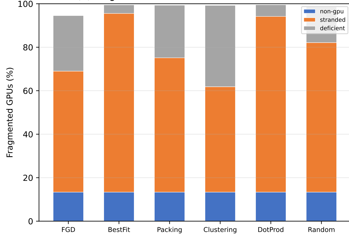
(d) Fragmentation breakdown into three causes
