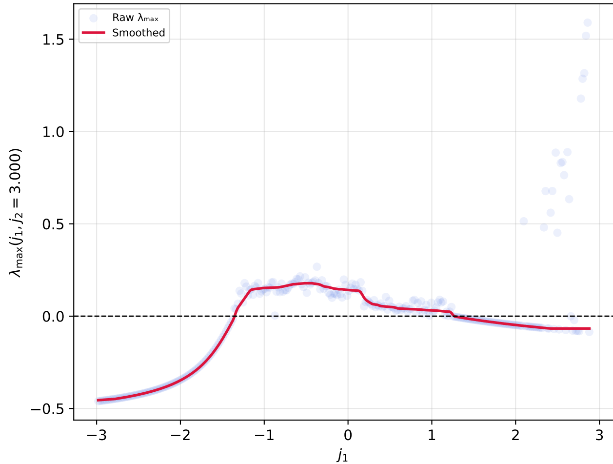
LLE Slice at j_2 = 3.000
