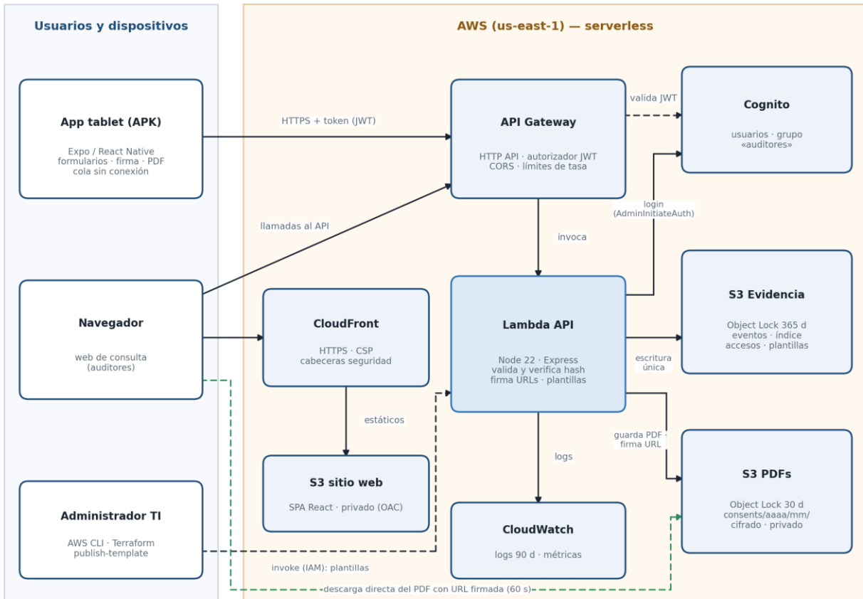
Figura 8. Arquitectura técnica de ACR Consentimiento Digital.
