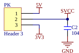
系统电源切换电路 5V or 3.3V
