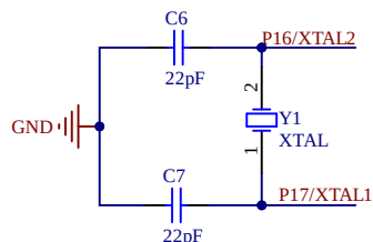
晶振电路 出厂默认无配置
