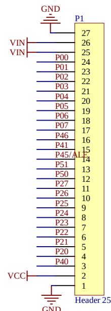
系统电源扩展接口
