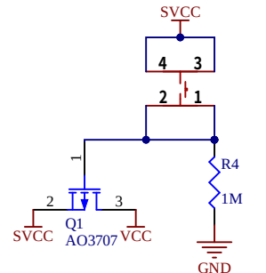
冷启动复位电路
