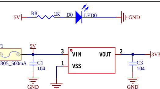
5V转3.3V电路及电源指示灯电路
