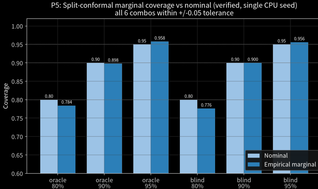
图 1 共形区间边际覆盖率：名义水平 vs held-out 实测（640 测试窗）。横轴为六个 (mode, \alpha ) 组合 (oracle/blind \times \alpha=0.2/0.1/0.05 )，纵轴为边际经验覆盖率；每对柱上方虚线标出名义水平 0.80/0.90/0.95，阴影带为 \pm 0.05 容差。所有柱落入容差带 (H1)。数据来源 reports7/v7_verification.json: coverage.* ，证据等级 verified，单 CPU 固定 seed 试点。
