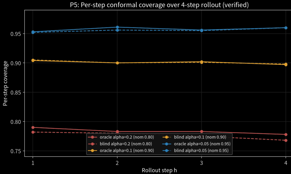
图 3 逐步（per-step）共形覆盖率随滚动步 h=1,2,3,4 的衰减曲线。横轴为自回归步 h ，纵轴为该步经验覆盖率；六条线对应 oracle/blind \times 80/90/95 三水平。可见低名义水平（blind 80%）随 h 单调下降（0.7831 \rightarrow 0.7672），高名义水平（blind 95%）末步反升至 0.9599——自回归误差累积在低带宽档更易暴露。数据来源 v7_verification.json: coverage.*.per_step ，verified，单 seed。
