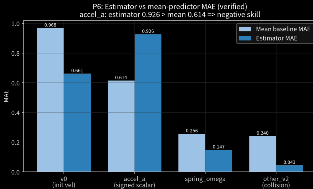
图 2 学习估计器 MAE（深）与训练集均值基线 MAE（浅）逐参数并列对照（横轴 v0/a/ \omega /v2，纵轴 MAE）。a 柱上深柱高于浅柱（0.926>0.614）即 skill 为负；其余三参数深柱低于浅柱即 skill 为正。数据来源 v7_verification.json: estimator_param_error.*.mae / mae_mean_predictor , verified, 单 seed。
