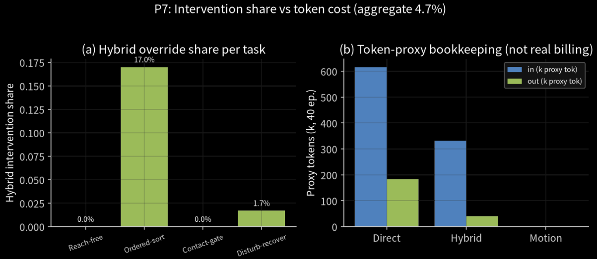
图 2 左: hybrid 在各任务上的接管率(横轴四任务, 纵轴 intervention_share 0-1), 集中在语义必需任务(ordered_sort 0.17、disturb_recover 0.017、纯接触 0); 右: 三模式 token 代理记账对比(direct 616k 入·182k 出 vs hybrid 331k·40k vs motion 0)。token 为按决策次数×固定单价的代理记账、非真实 API 计费, 只作方向性对比。数据来源 embodied_hybrid_demo.json: by_task.*.intervention_rate / aggregate.*.tokens_*_proxy_total , cpu-proto, 单 seed。
