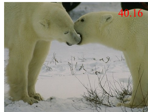
DACA-IR(ours)
