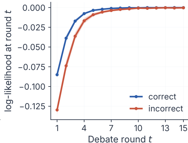
LL: gap collapses
