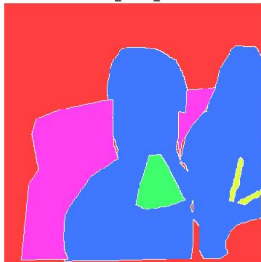
true_mask_val
