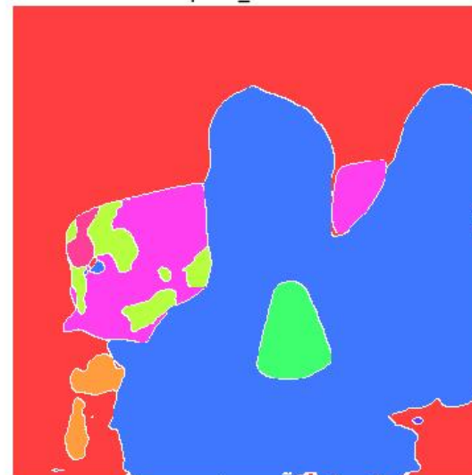
pred_mask
