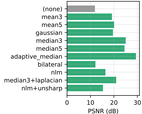
saltpepper_20
