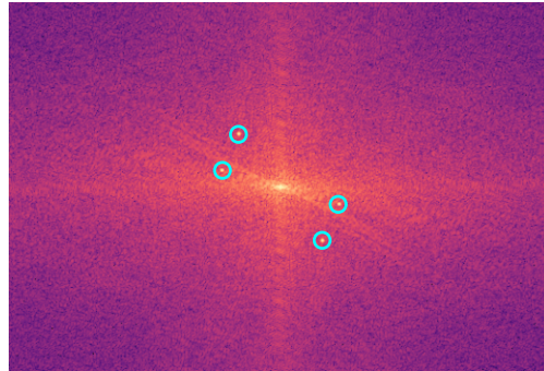
\log |F(u,v)| (Hann)
