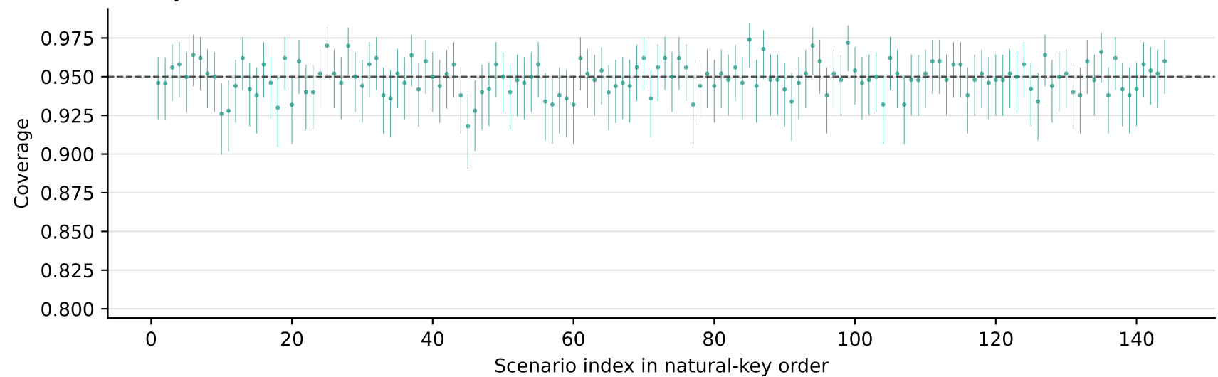
DML-style IVQR
