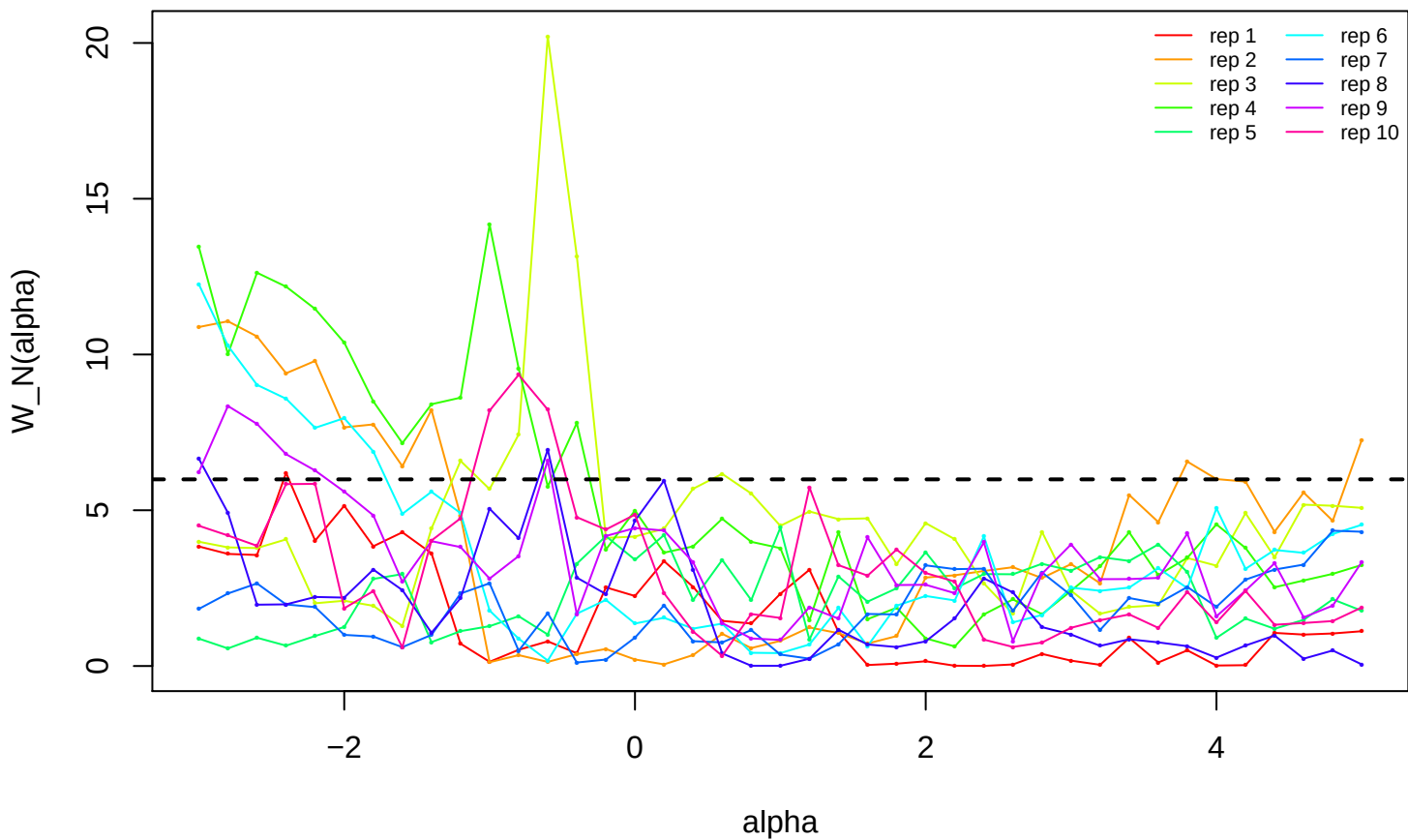
DML-IVQR tau = 0.10 kappa = 0.10, n = 500
