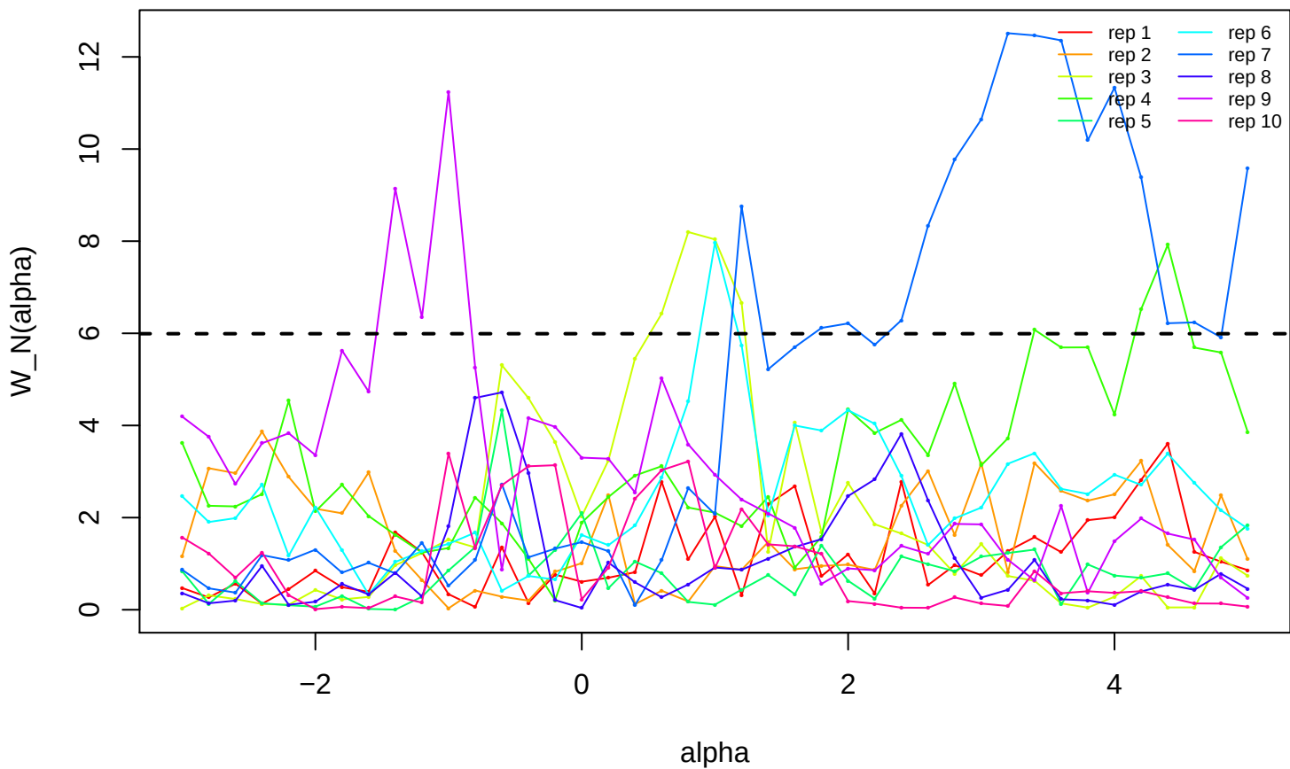
Oracle-GMM tau = 0.10 kappa = 0.10, n = 500
