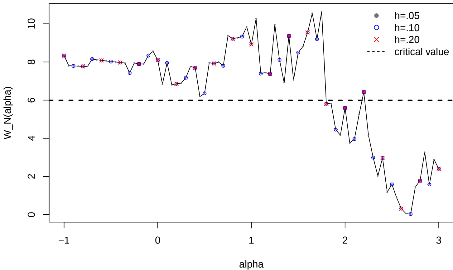
simple rep 1 DML-IVQR tau 0.90
