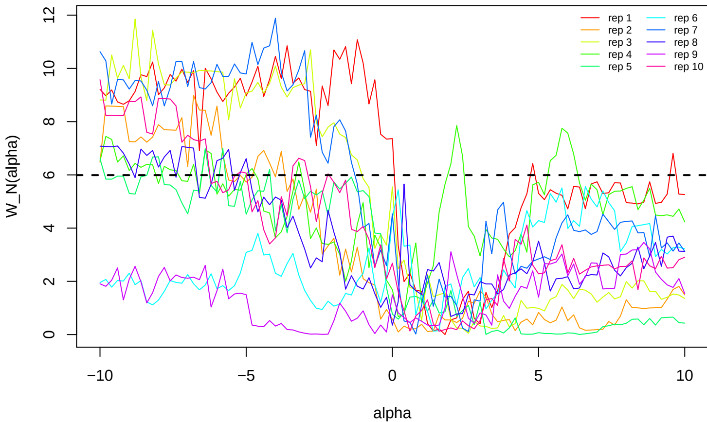
DML-IVQR tau = 0.50 [-10,10]
