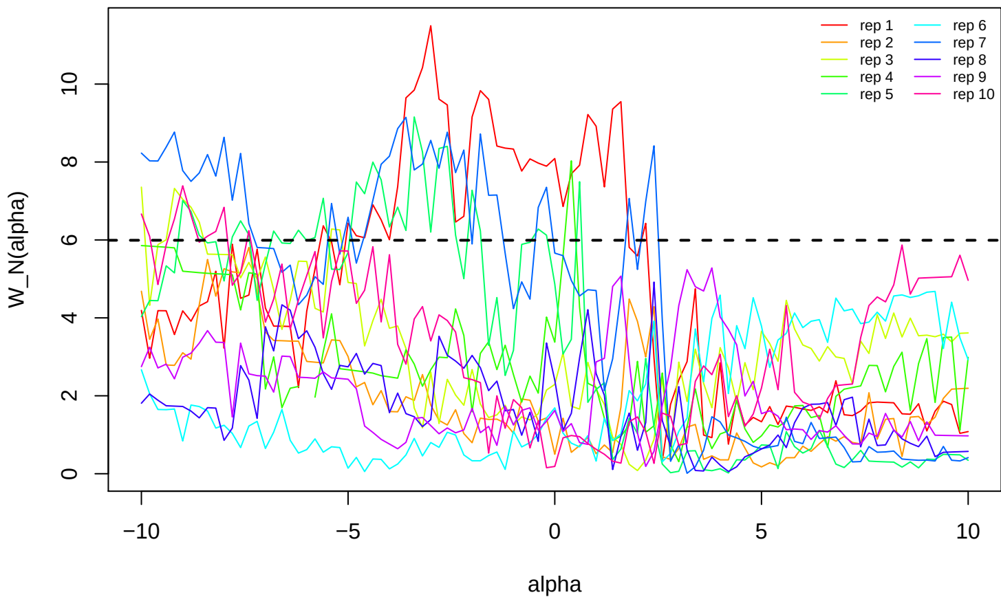
DML-IVQR tau = 0.90 [-10,10]
